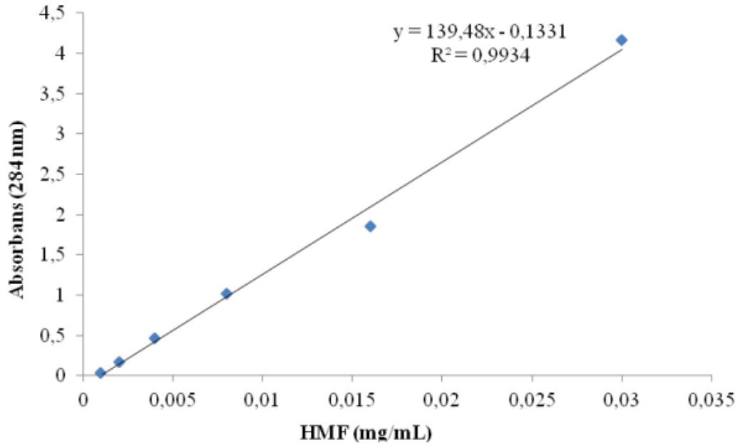
Şekil 3-10 HMF kalibrasyon eğrisi
