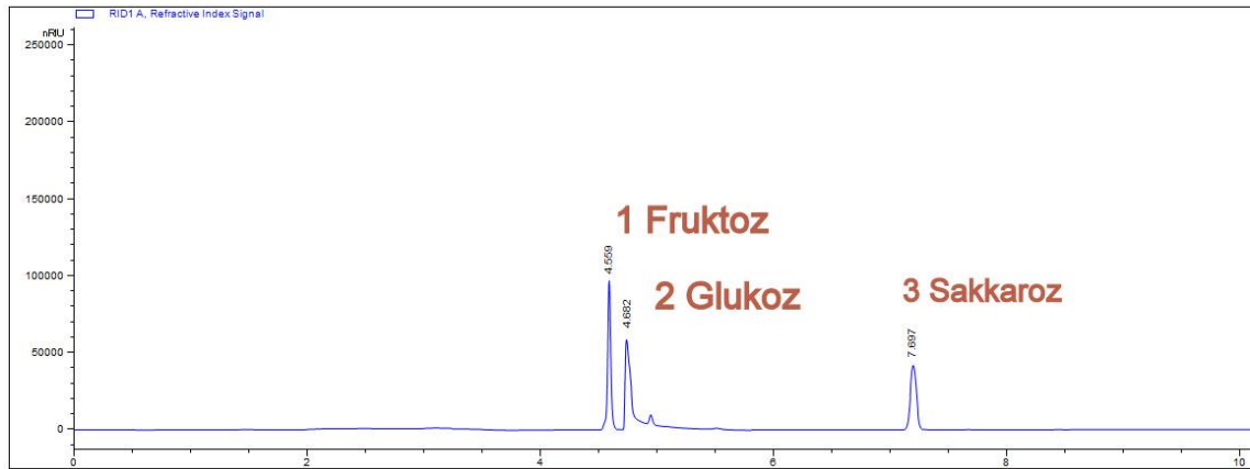
Şekil 3-9 Standart örneklerin diyagramı
