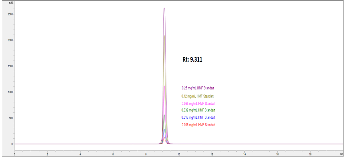
Şekil 3-11 HMF standart diyagramı
