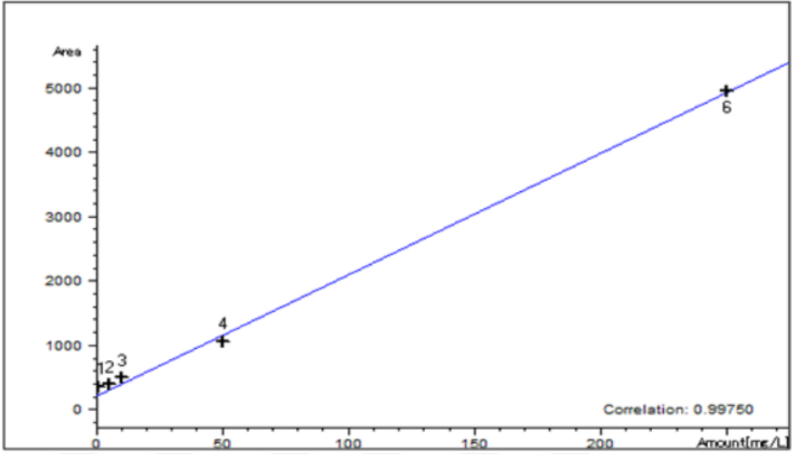
Şekil 3-4 Pyridoxine (B6) standardı kalibrasyon eğrisi
