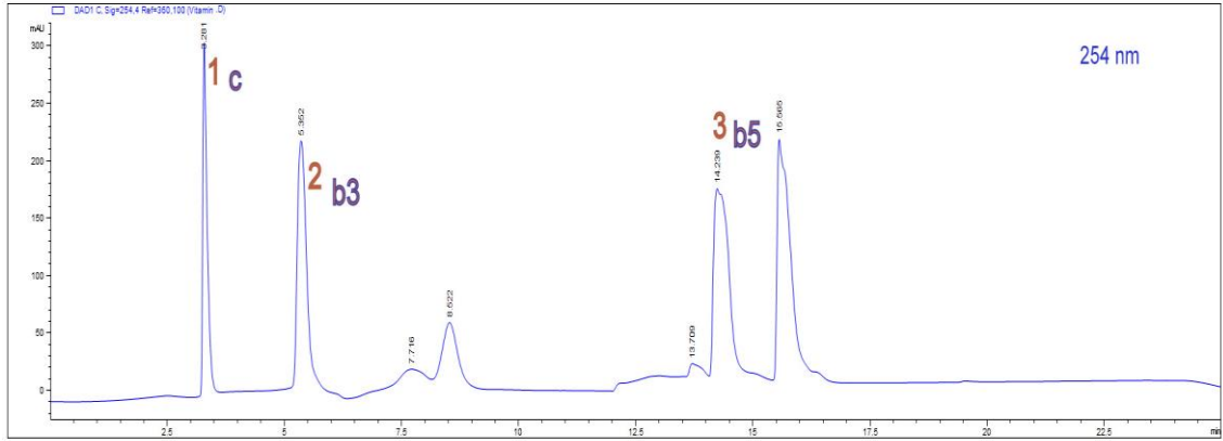
Şekil 3-7 C, B3 ve B5 vitamini standart diyagramı
