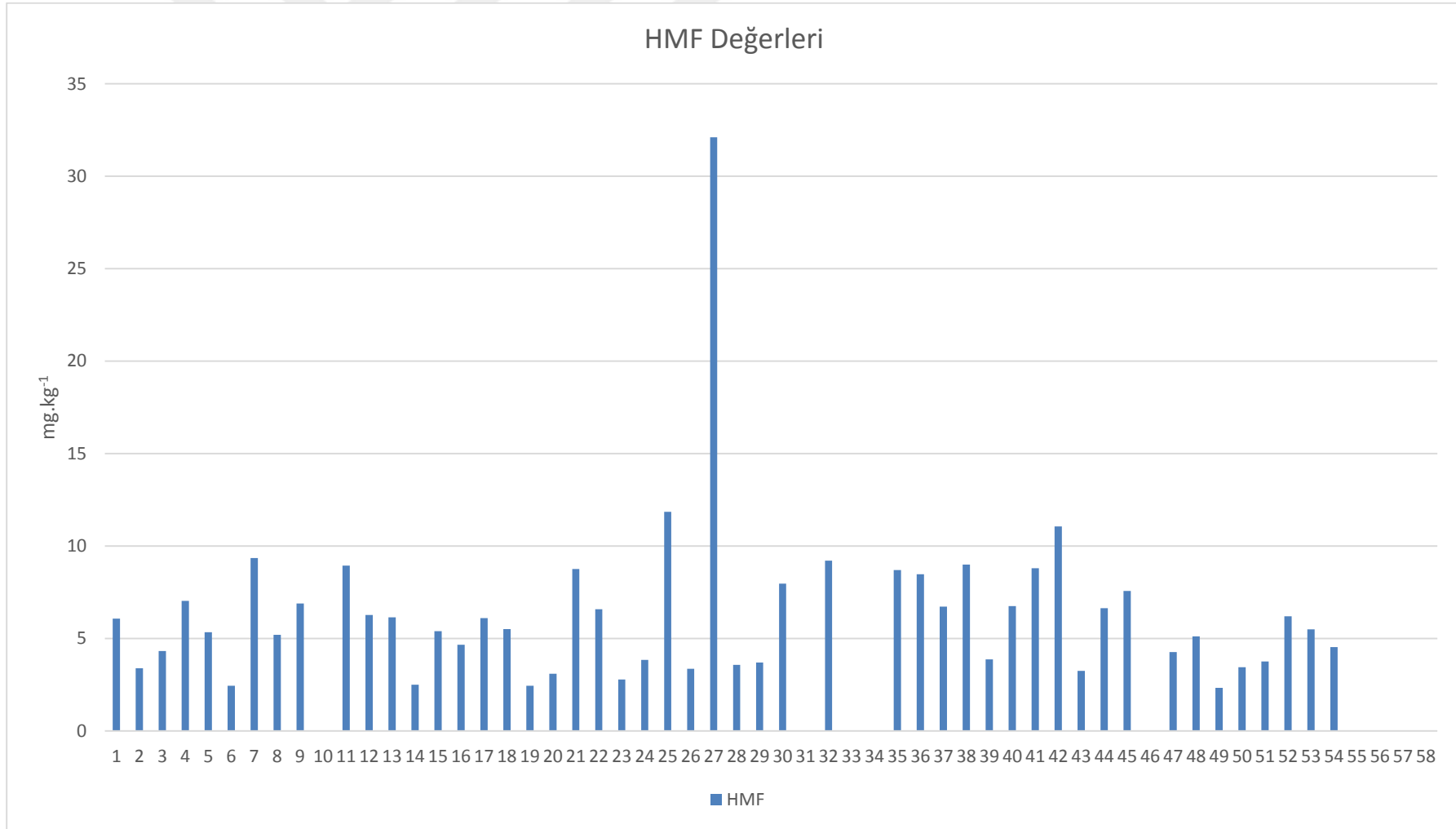
Şekil 4-7 Numunelerin HMF değerlerini gösterir grafik
