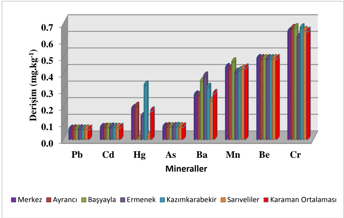
Şekil 4-1 İlçeler Pb, Cd, Hg, As, Ba, Mn, Be ve Cr değerleri
