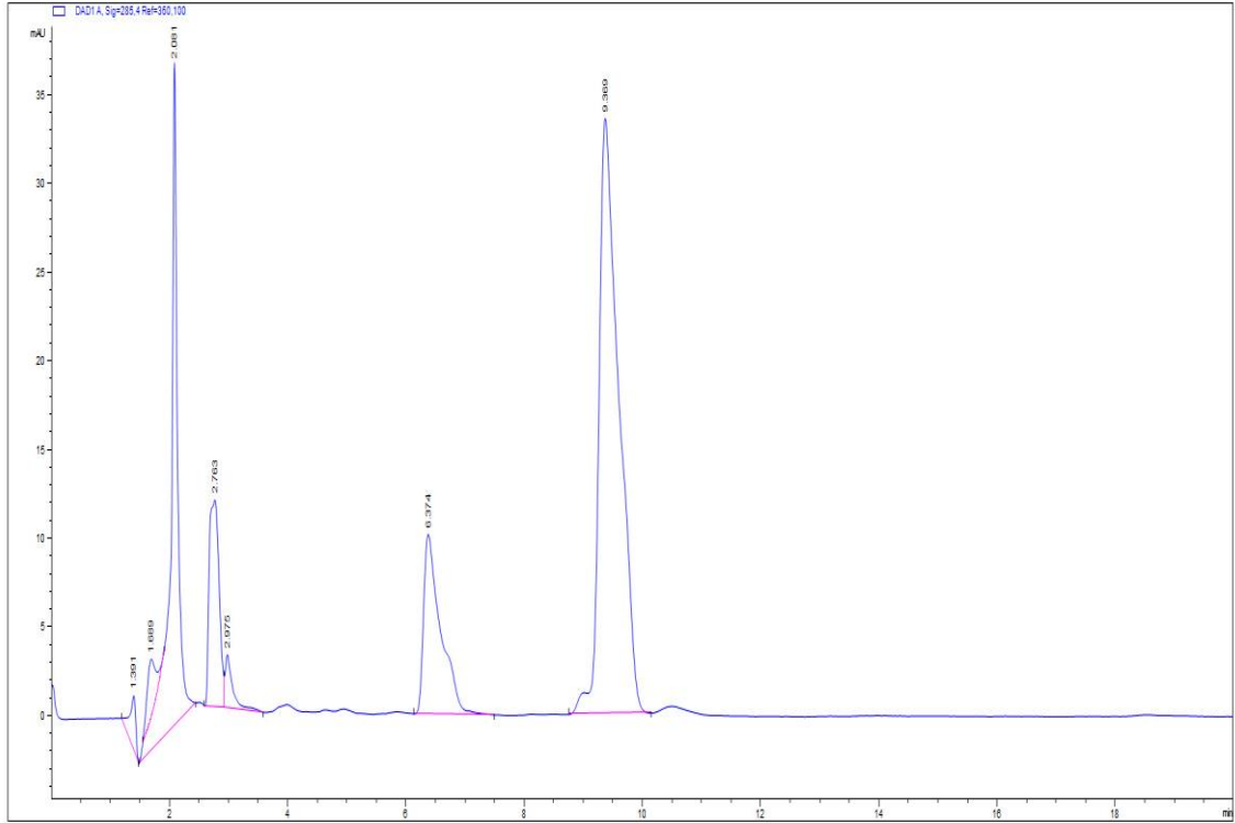
Şekil 3-12 Numuneye ait diyagram
