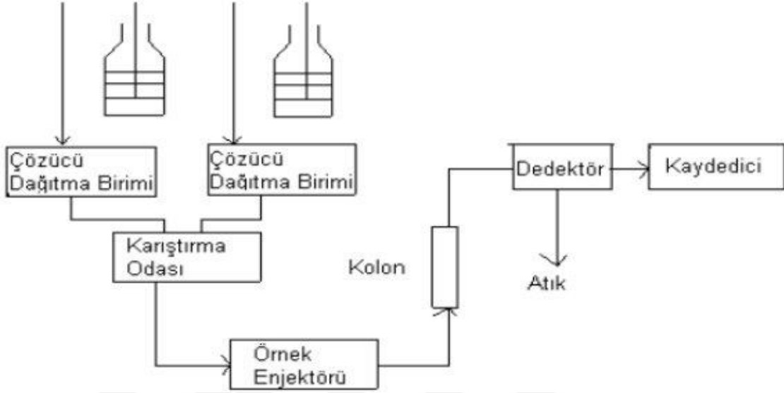
Şekil 2-2 HPLC cihazı çalışma prensibi
