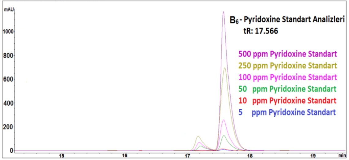
Şekil 3-6 Pyridoxine (B6) vitamininin ara stok çözelti kromatogramları
