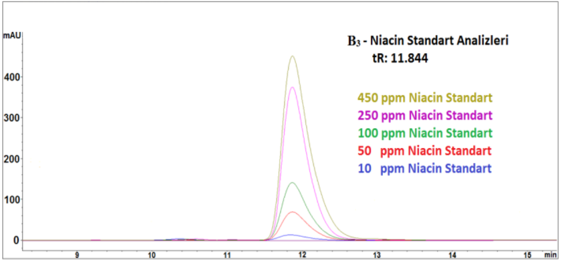
Şekil 3-5 Niacin (B3) vitamininin ara stok çözelti kromatogramları
