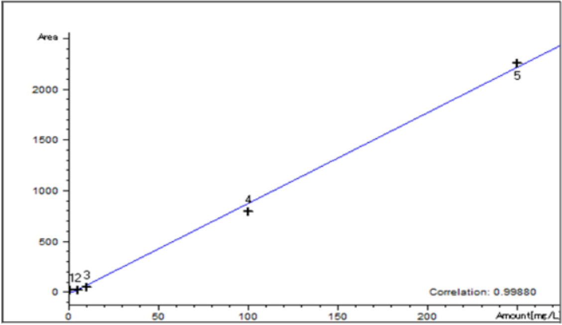
Şekil 3-2 Riboflavin (B2) standardı kalibrasyon eğrisi
