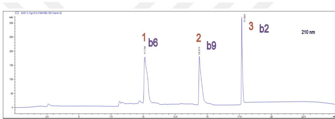
Şekil 3-8 B2, B6 ve B9 vitamini standart diyagramı
