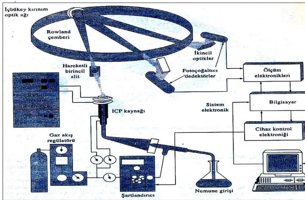
Şekil 2-1 ICP-OES spektrofotometre cihaz şeması
