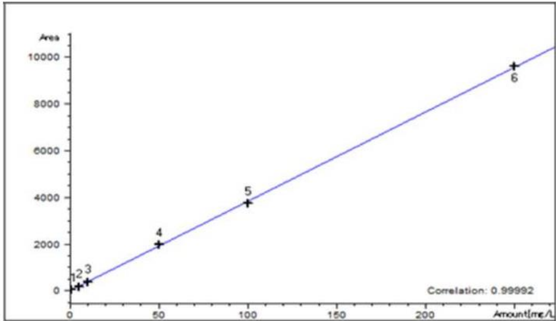
Şekil 3-3 Niasin (B3) standardı kalibrasyon eğrisi
