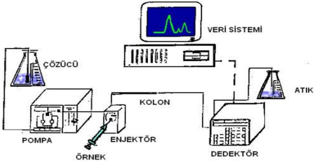
Şekil 2-3 HPLC cihazının genel gösterimi
