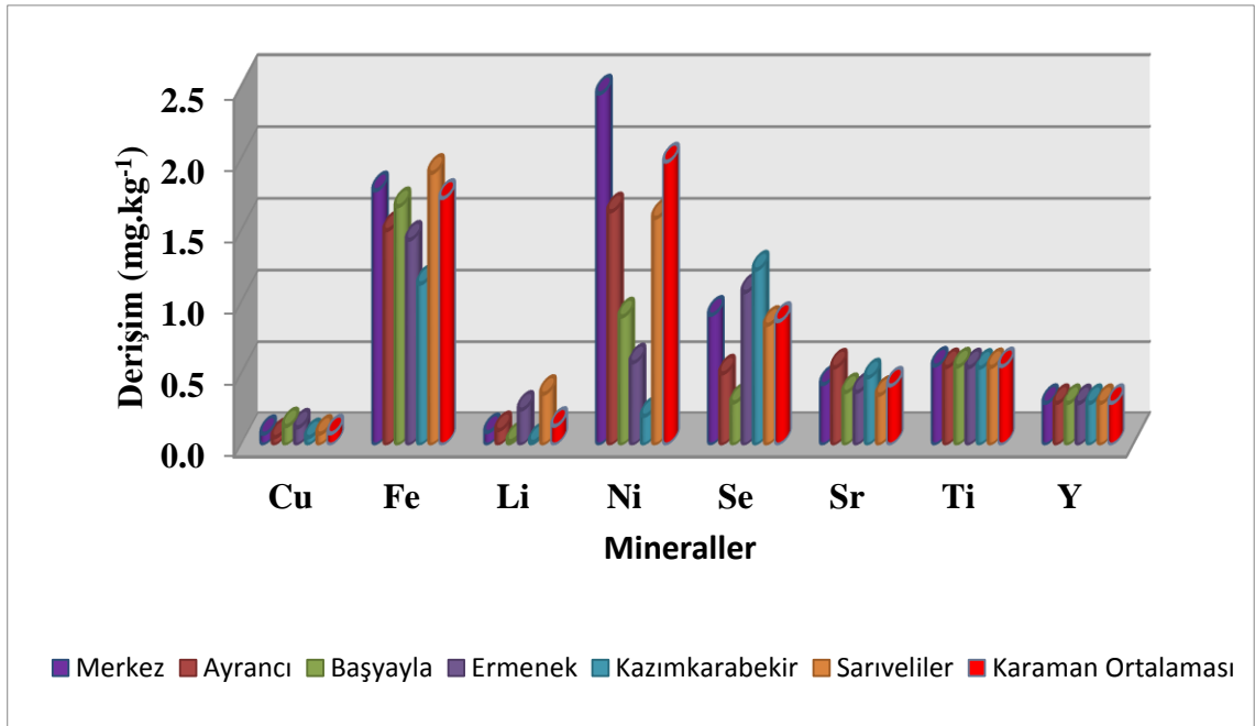
Şekil 4-2 İlçeler Cu, Fe, Li, Ni, Se, Sr, Ti ve Y değerleri
