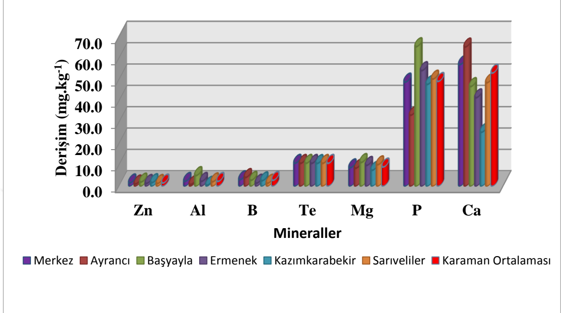
Şekil 4-3 İlçeler Zn, Al, B, Te, Mg, P ve Ca değerleri
