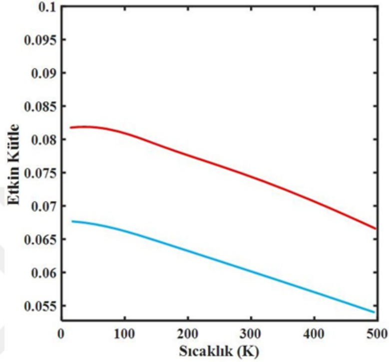
Şekil 3.4. GaAs için elektron ve boşluk etkin kütlelerinin sıcaklıkla değişimi. Altta ki eğri elektron için, üstteki eğri boşluk etkin külesini gösterir.
