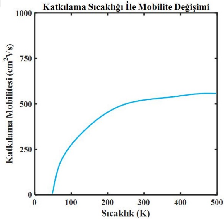
Şekil 3.11. Katkı ile sıcaklığın mobilite ile değişimi.
