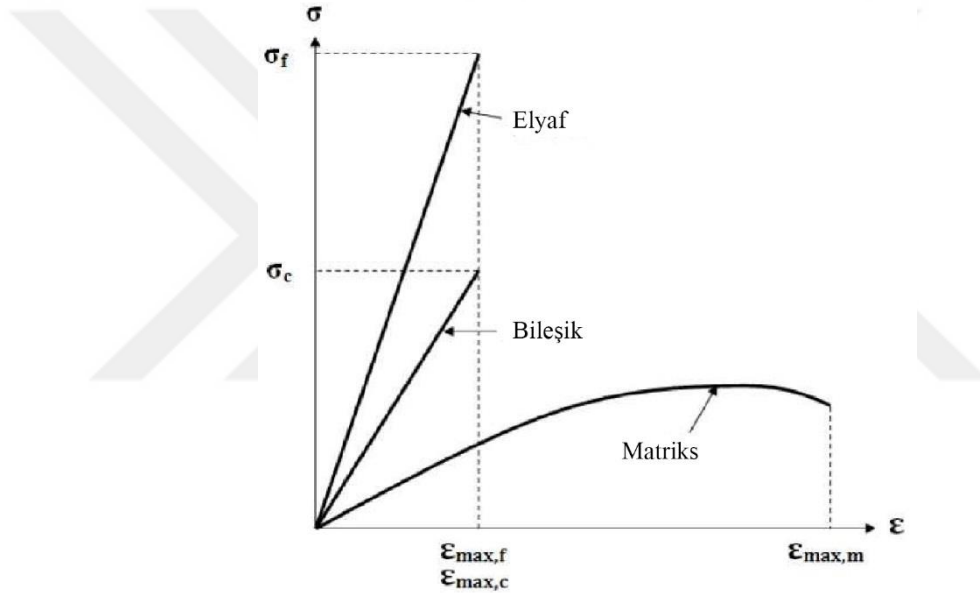
Şekil 3.3. CTP kompozit ve bileşenleri için gerilme-birim şekil değiştirme ilişkisi [20].
