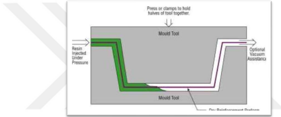
Şekil 5.7. Reçine transfer kalıplama işlemi/ çizim [33].
