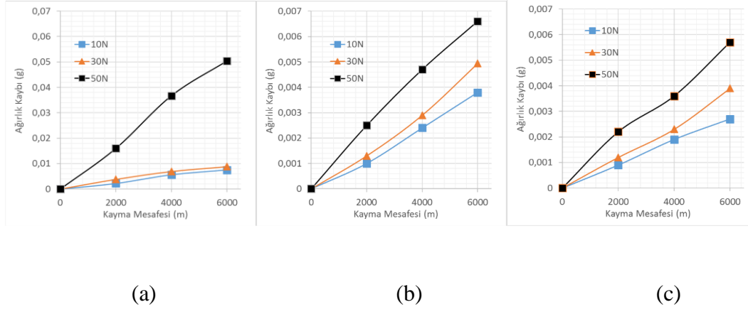
Şekil 8.5. % 3.5 NaCl içeren korozif ortamda (a) S355JR , (b) kalın kesitli ve (c) ince kesitli CTP kompozitlerin ağırlık kaybı-kayma mesafesi grafikleri.
