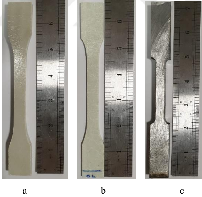
Şekil 7.4. İşlenmiş (a) kalın kesitli CTP, (b) ince kesitli CTP ve (c) çelik çekme deney numunelerinin görünümü
