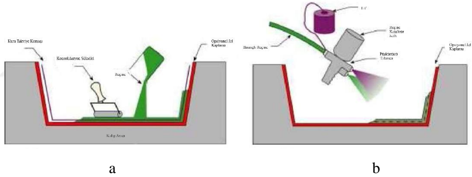
Şekil 5.1. Yarı otomatik (a) Elle Döşeme ve (b) püskürtme işlemi [33].
