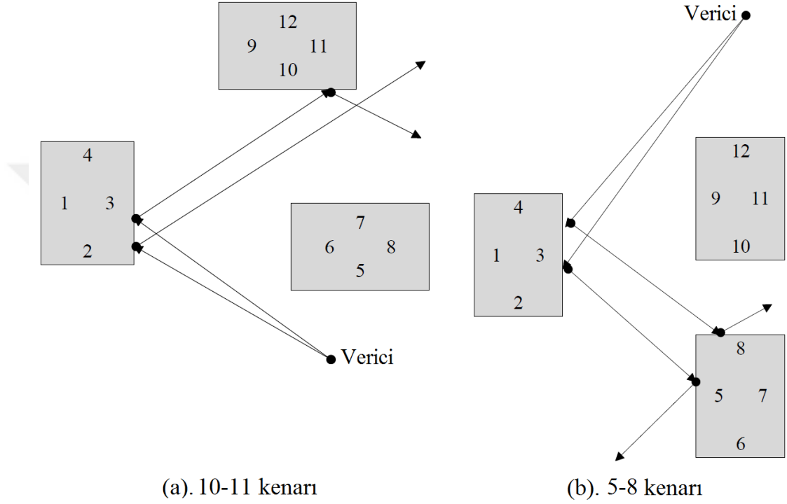
Şekil 3.1. Kırınım kenarlarını tanımlayan bitişik ışınlar.
