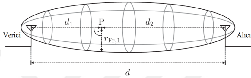
Şekil 2.2. Birinci Fresnel bölgesi.
