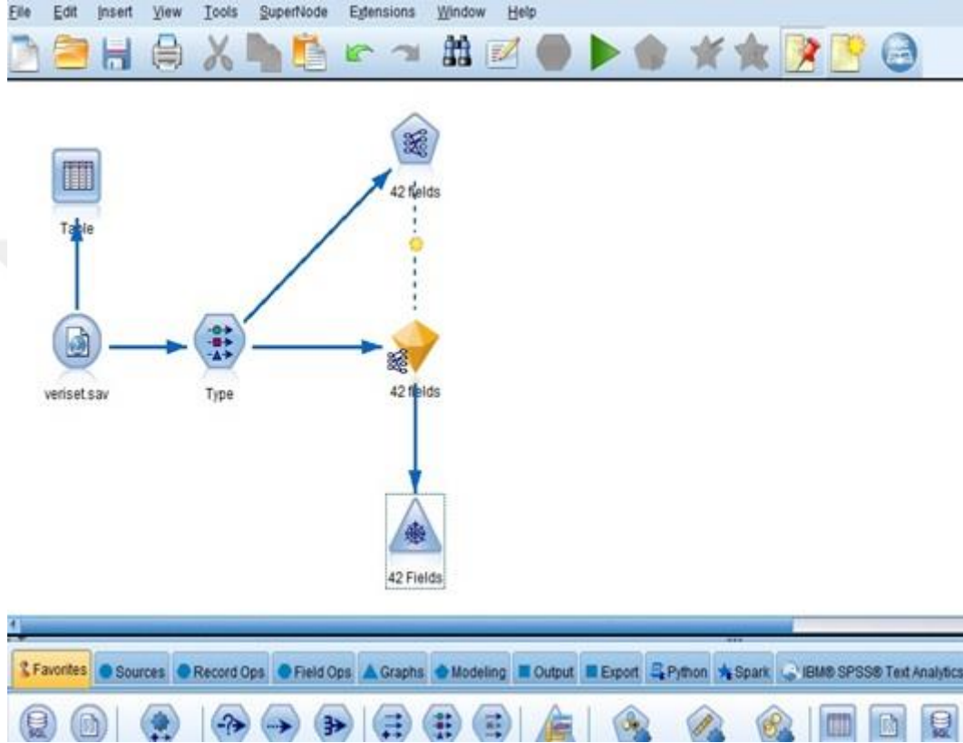
Şekil 5.1: Algoritma Aşamaları
