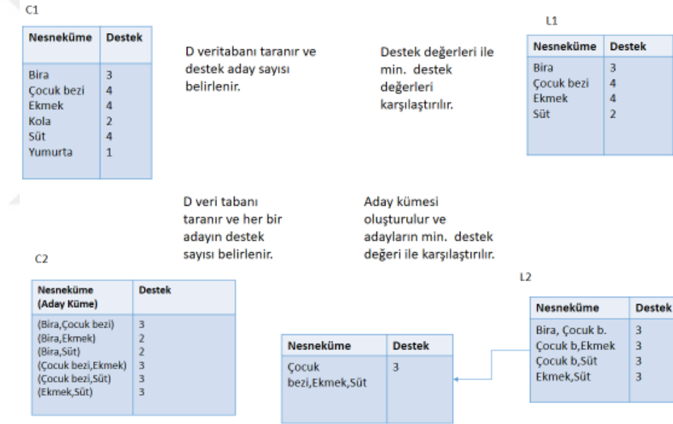
Şekil 4.1: Apriori Algoritmasının Adımları
