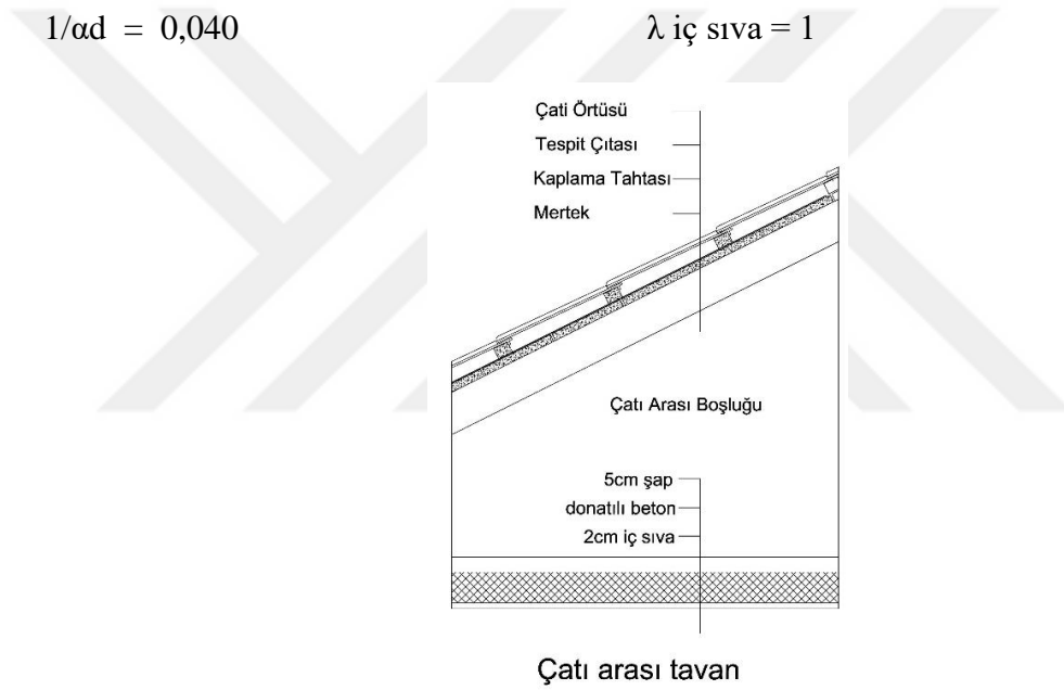
Sekil A.2: Çatı arası tavan detayı
