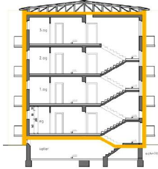
Şekil 1.6: Yeni termal bina kabuğunun kesiti [Url-2]
