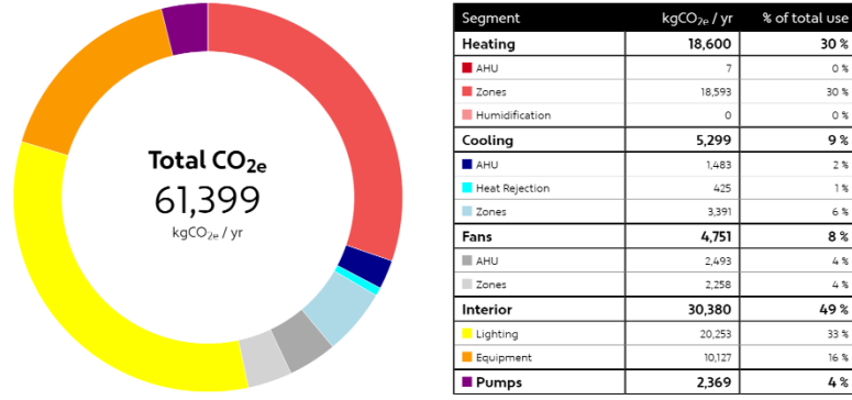
Şekil 4.10: S6 alternatifi CO2 emisyonu miktarı.
