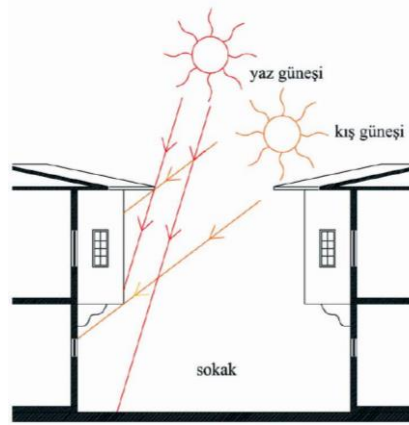
Sekil C.4: Kaleiçi yerlesmesinde saçak ve çıkmaların güneş ısınlarının gelis açısına göre boyutlandırılması (Akın, 2001)
