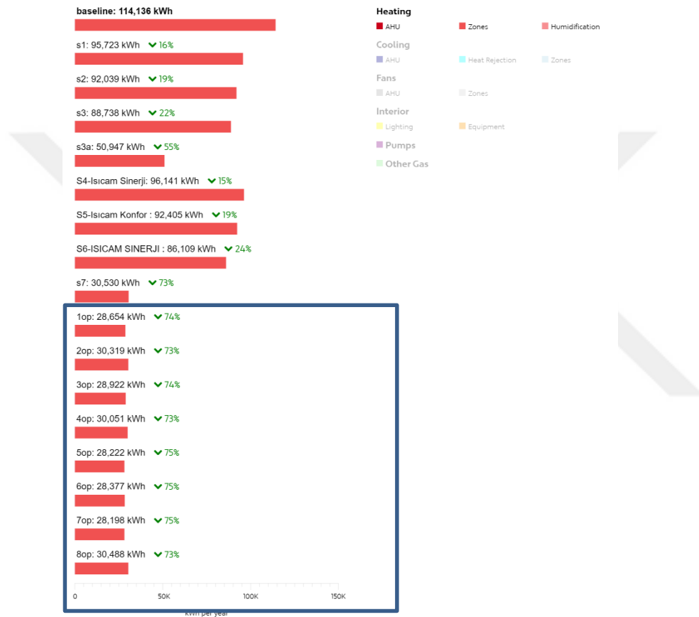
Şekil 4.6: Cephe tasarım alternatiflerinin yıllık toplam ısıtma yükü
