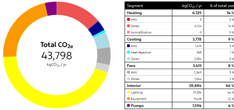
Şekil 4.12: 6OP(S13) alternatifinin CO2 emisyonu miktarı.
