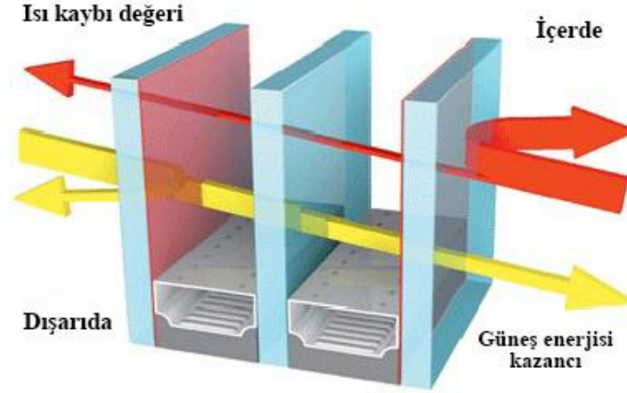
Şekil 2.9: Üçlü Şeffaf Cam için Enerji Dağıtımı [Url-8]
