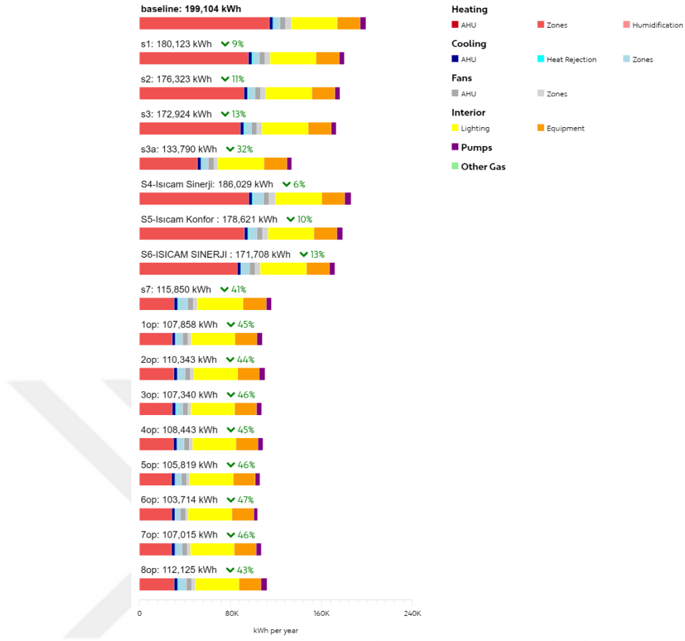
Şekil 4.4: Geliştirilen alternatiflerin sonrası yapının ısıtma soğutma yükleri
