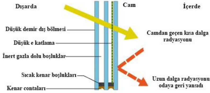
Şekil 2.10: Low-e Üçlü Şeffaf Cam için Enerji Dağıtımı [Url-9]
