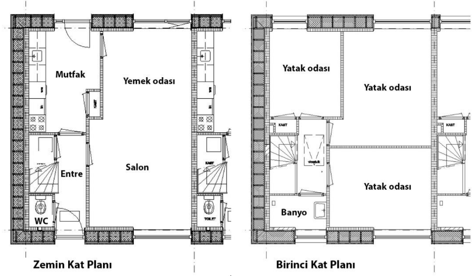
Şekil 1.16: Yenilenmiş binanın kat planı değişiklikleri[14].
