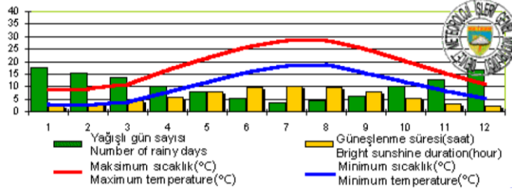
Şekil 2.18: İstanbul iline ait yıllık sıcaklık, yağışlı gün sayısı ve güneşlenme süreleri [53] .
