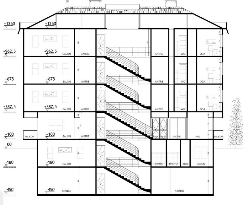
Şekil 3.8: Örnek Binanın A-A kesidi
