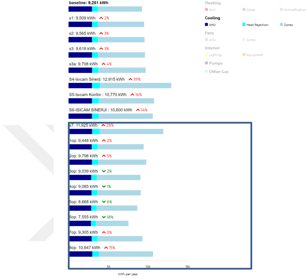
Şekil 4.7: Cephe tasarım alternatiflerinin yıllık toplam Soğutma yükü
