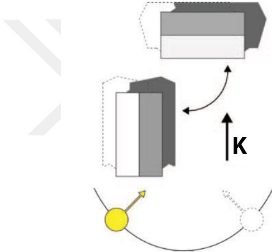
Şekil 2.3: Günün çeşitli saatlerinde güneşin konumu [18]
