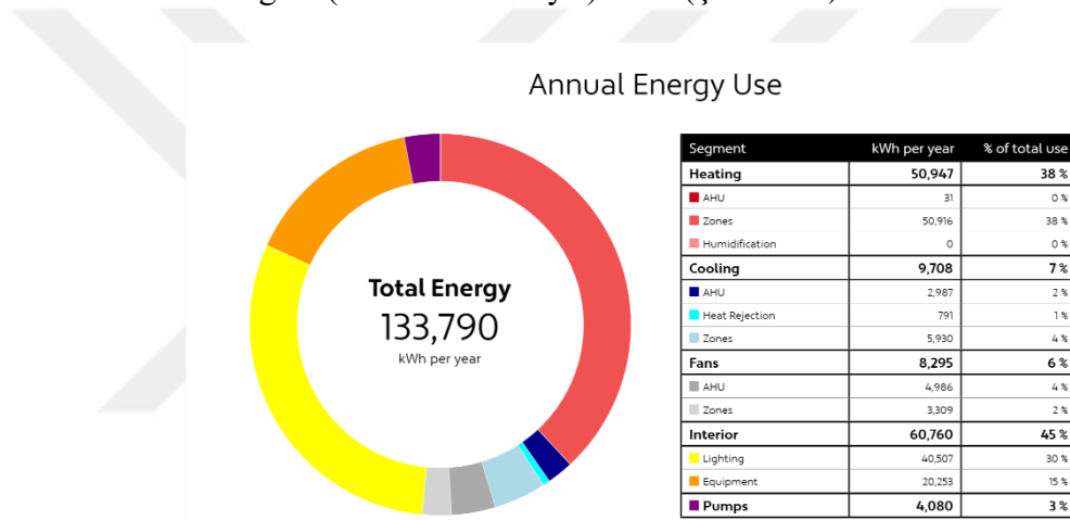
Şekil 4.1: S3A Enerji Tüketiminin Değerleri
