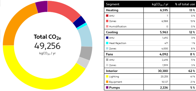
Şekil 4.11: S7 alternatifi CO2 emisyonu miktarı.
