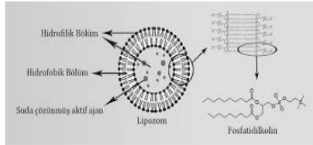
Şekil 3.13: Lipozomun yapısı
