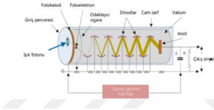
Şekil 4.5: Foton çoğaltıcı tübün yapısı
