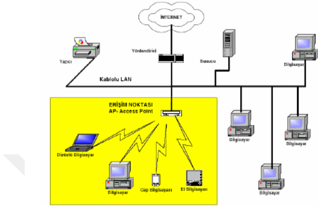
Şekil 2.5.1.1 : WLAN çalışma modeli Kaynak : (Yılmaz H., 2007)
