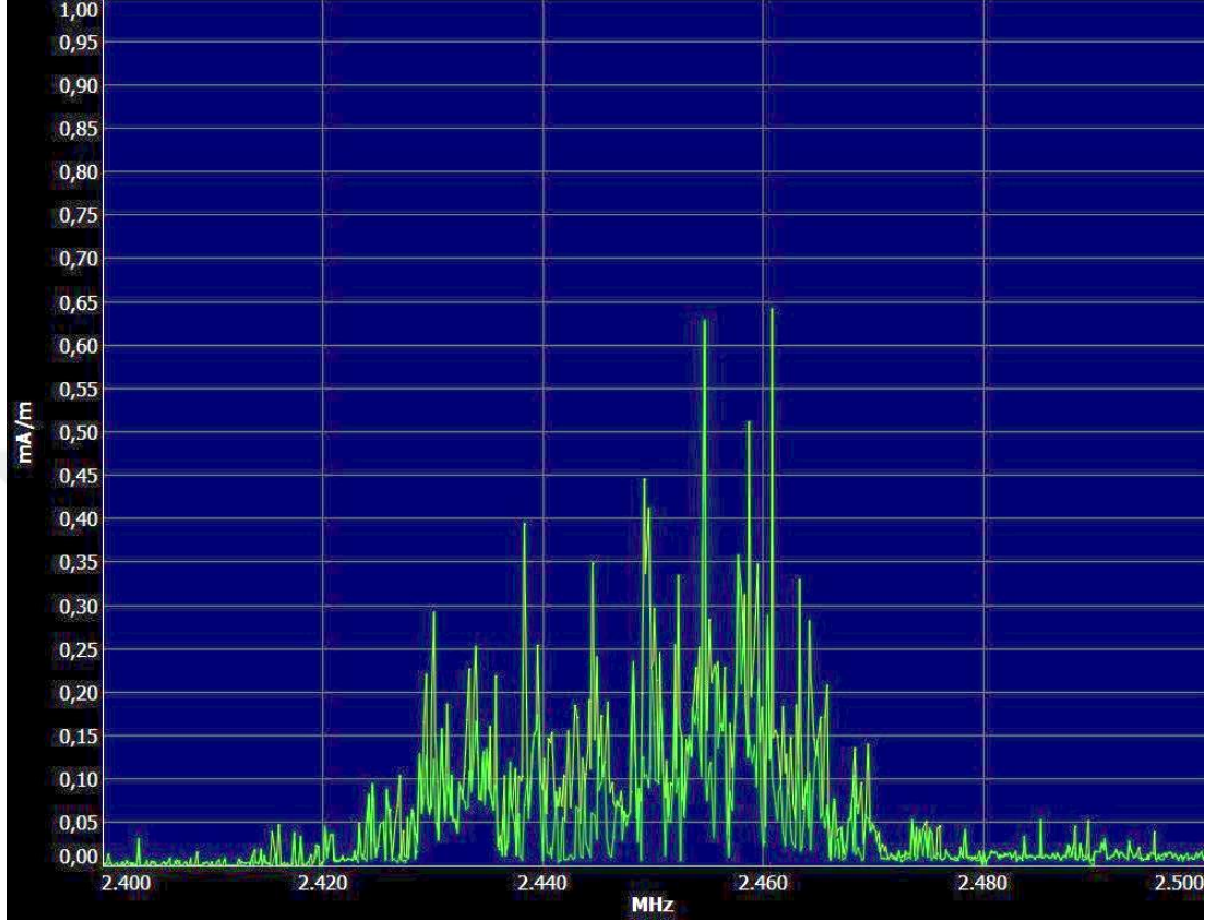
Şekil 6.2.9 : 2 cihaz modemle veri transferi hâlindeyken, modeme 4 metre uzaklıkta ölçülen Manyetik Alan'ın, Wi-Fi frekanslarındaki dağılımı
