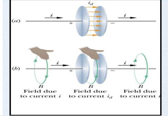
Şekil 2.6.1.1 : Amperè - Maxwell denkleminin gösterimi Kaynak : Url-1
