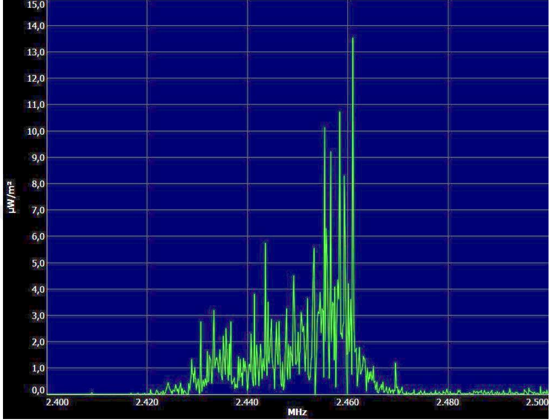
Şekil 6.2.1 : 1 cihaz modemle veri transferi hâlindeyken, modeme 4 metre uzaklıkta ölçülen Güç Yoğunluğu'nun, Wi-Fi frekanslarındaki dağılımı
