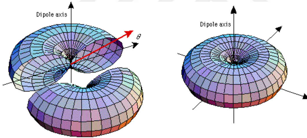
Şekil 5.1.2 : Dikey kutuplu çok yönlü anten ışınım modeli
