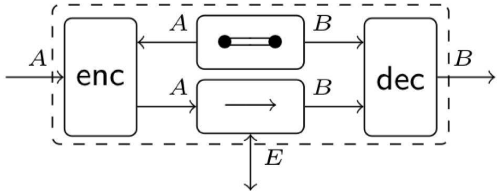
Şekil 3.6: Kanala Uygulanan Şifreleme Protokolü (enc, dec) - \rightarrow ve Tuşu \bullet == \bullet
