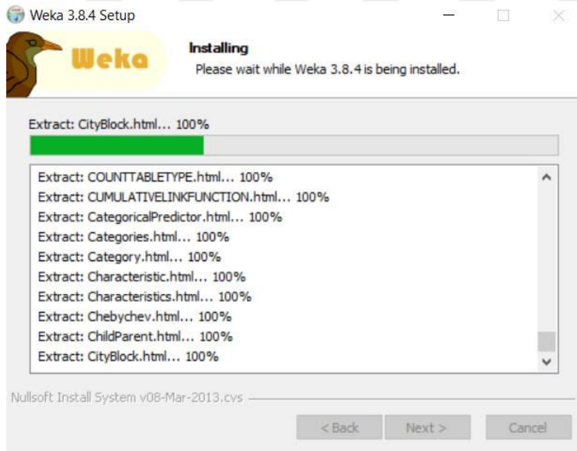
Şekil 3.2.2.1 Weka Kurulumu
