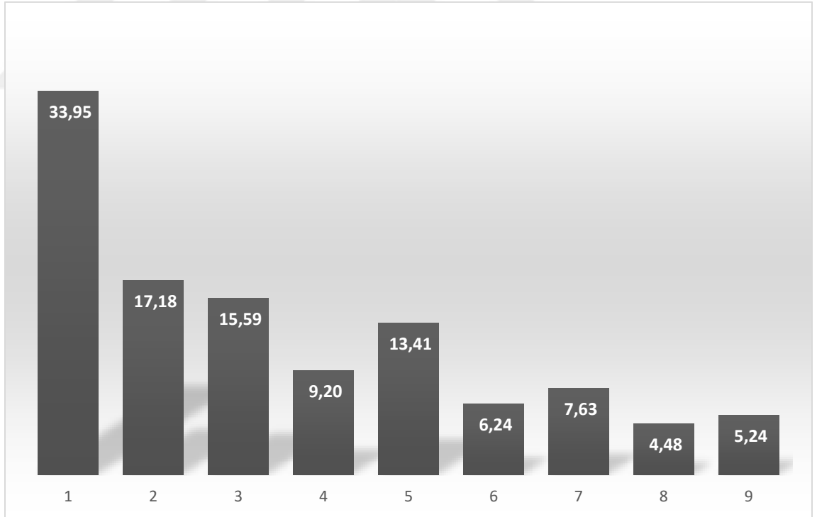
Grafik 4.1. Benford Yasası Gözlem Alanı Verilerinin Dağılımı
