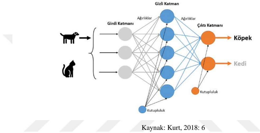
Şekil 13. Evrişimli Sinir Ağının Kavramsal Örneği
