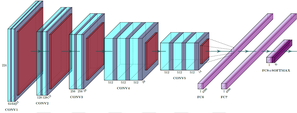
Şekil 14. VGG-16 Mimarisi
