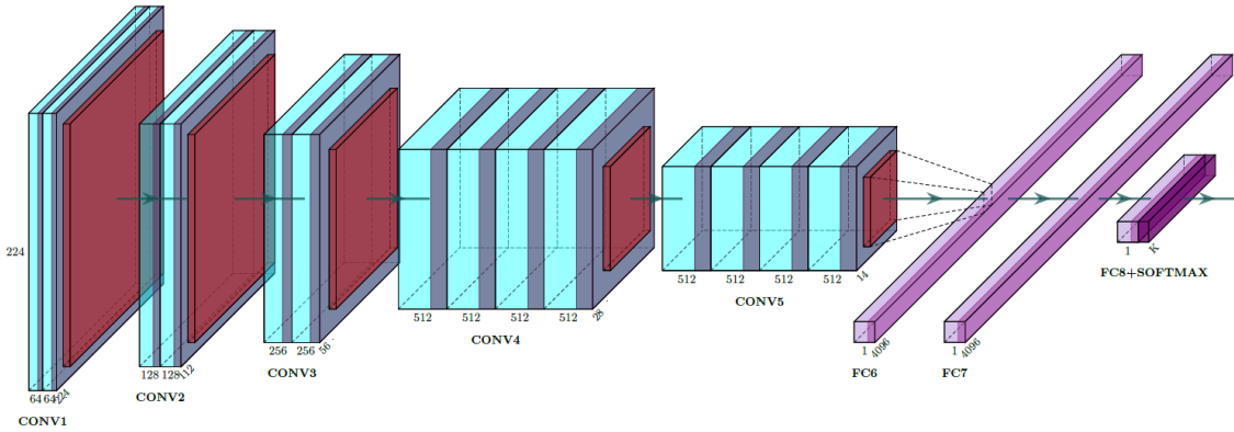
Şekil 15. VGG-19 Mimarisi
