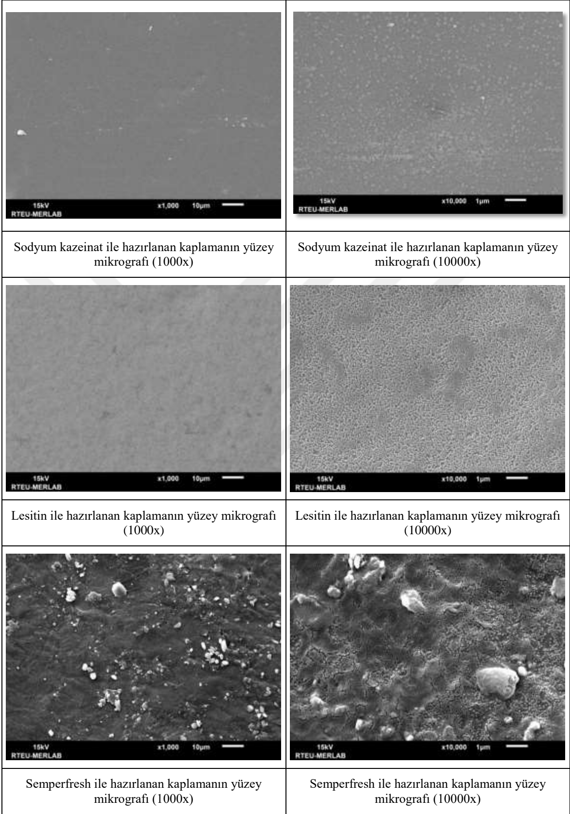
Şekil 3.16. Kaplamaların yüzey mikrografları
