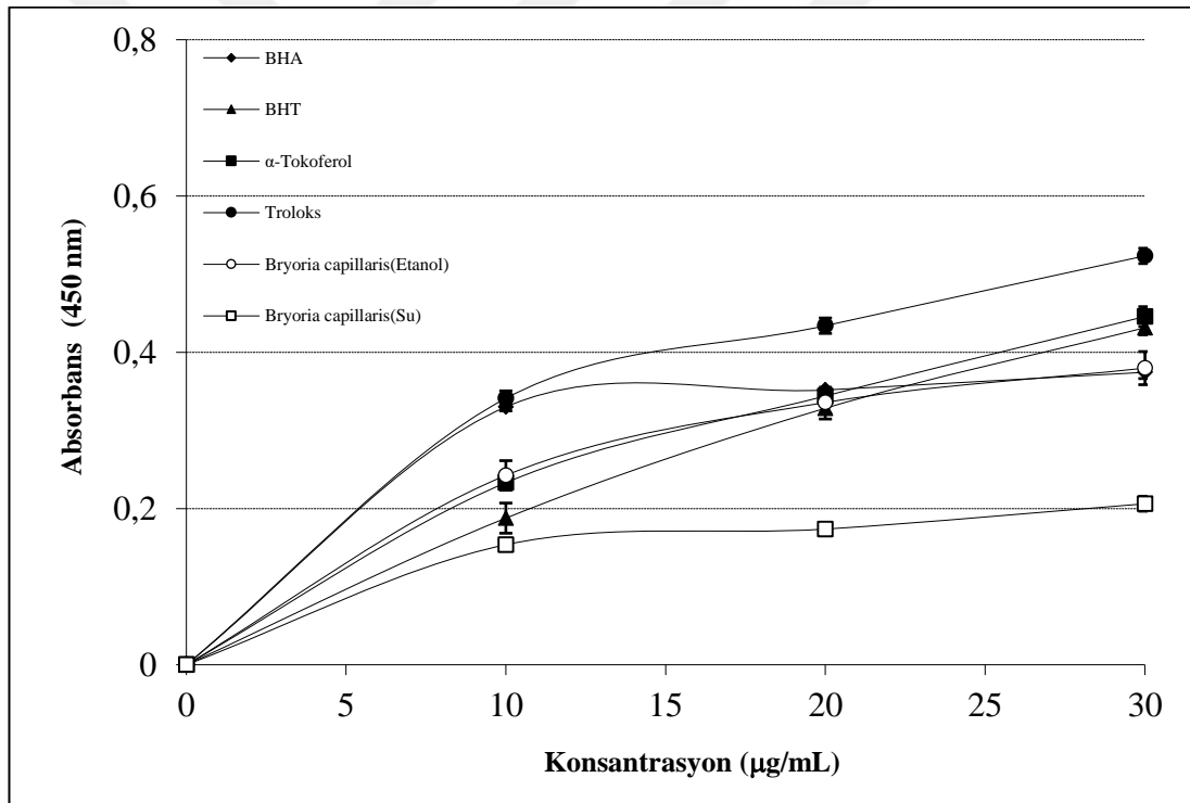
Şekil 3.3. Liken Bryoria capillaris etanol ve su ekstraktlarının farklı konsantrasyonlardaki (10-30 \mu\text{g}/\text{mL} ) çözeltileri ve standart antioksidanların (BHA, BHT, \alpha -tokoferol ve troloks) \text{Cu}^{2+} - \text{Cu}^+ indirgeme kapasitesi grafiği
