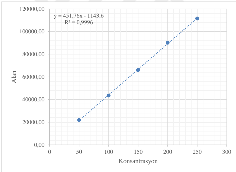
Şekil 2.9. Kalibrasyon eğrisi
