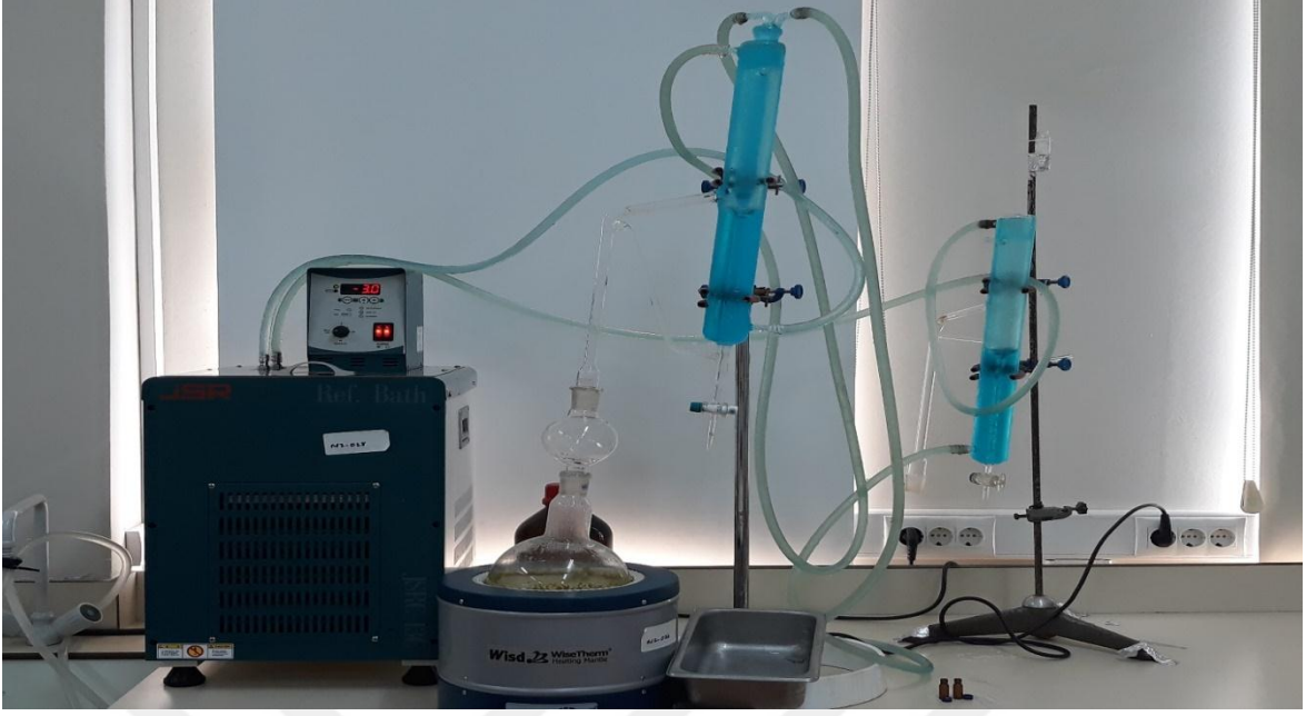
Şekil 2.3. Çalışmada kullanılan Clevenger düzeneği
