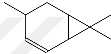
4-Karen(PcÇ)
