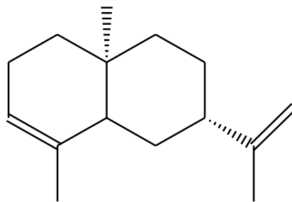
Selinenen(PcÇ)
