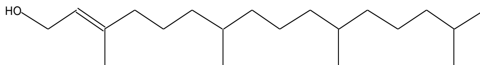
Fitol( PcÇ )
