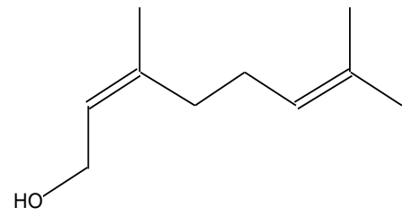
Cis-Geraniol( PcÇ )
