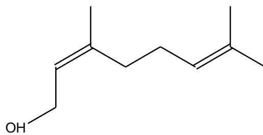
Nerol(PcY)
