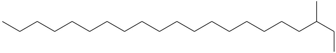
3-Metilheneikosan( PcC )
