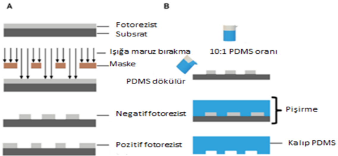
Şekil 3.1. Mikroakışkan ekipmanın üretiminde kullanılan litografi ve yumuşak litografi işlemleri (Keçili, 2019).
