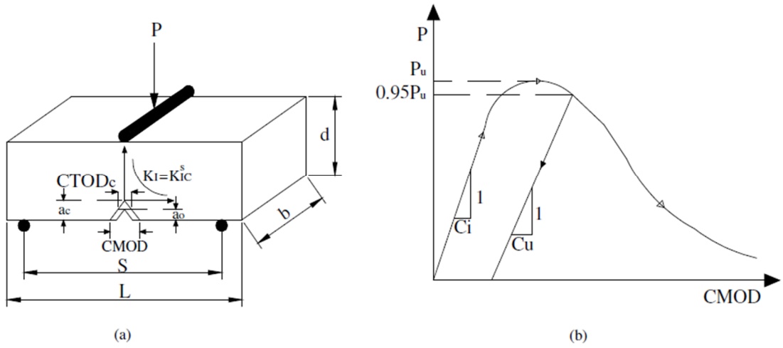
Şekil 2.6. İki parametrelili kırılma modeli. a) çentikli üç noktali eğilme numunesi, b) tipik bir P-CMOD diyagramı.
