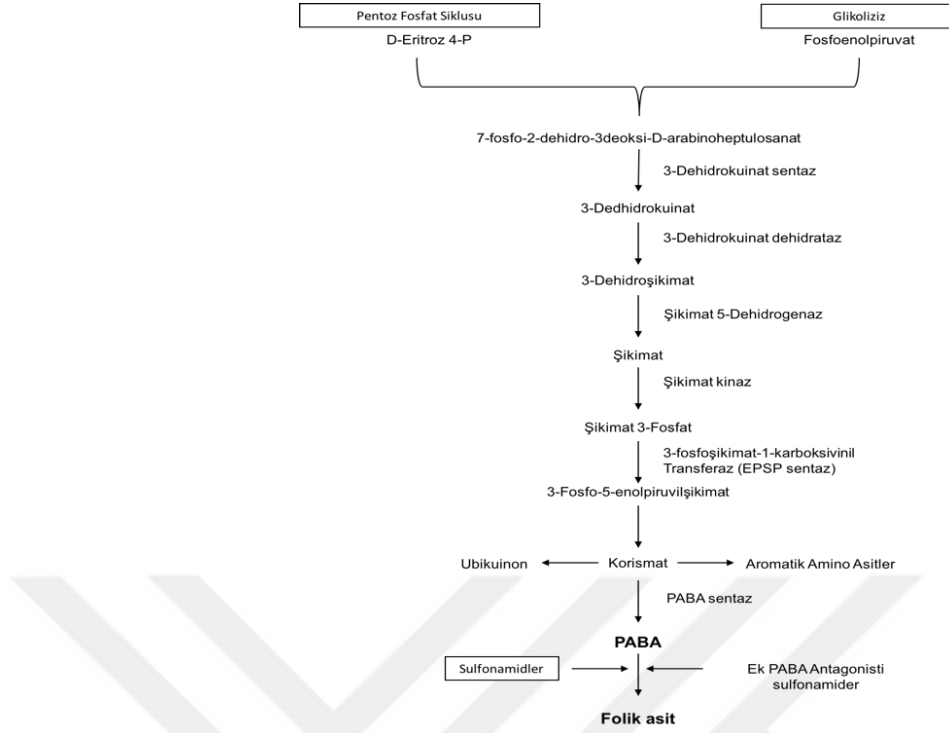
Şekil 1.1. Aromatik aminoasit biyosentez yolağı.
