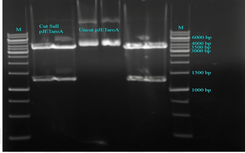
Şekil 3.3. pJETaroA vektörünün Sall restriksiyon enzimi ile kesimi sonrası jel görüntüsü (M: 1kb DNA Ladder).
