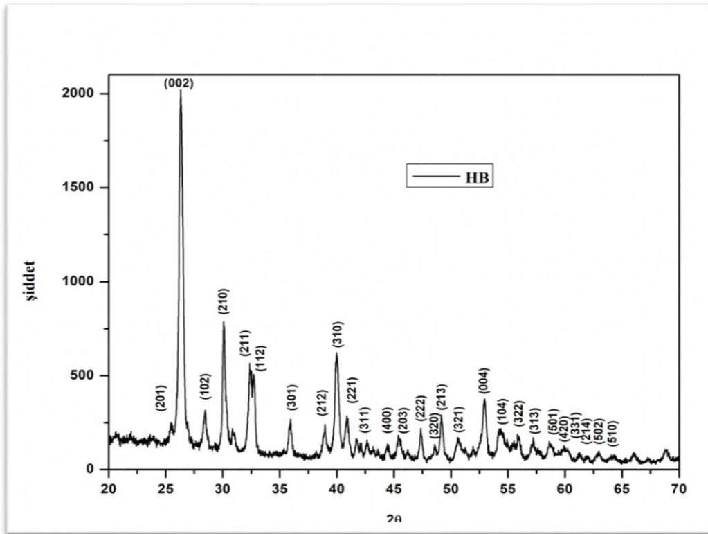
Şekil 5.1. HAp bileşiminin XRD difraksiyon pikleri
