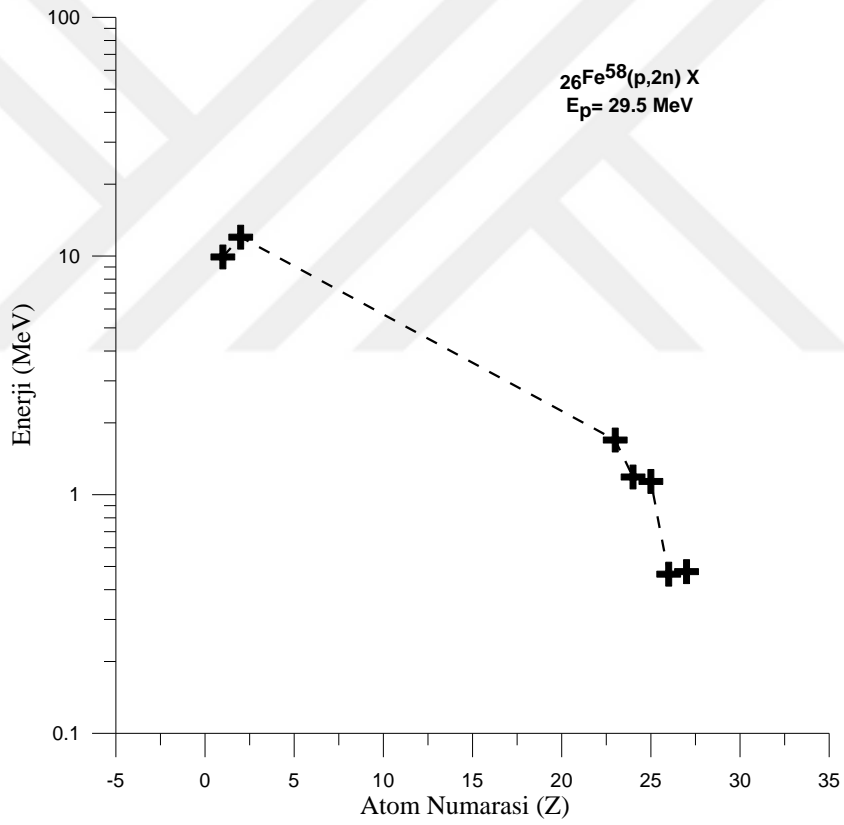
Şekil 4.43. Demir elementinin 29,5 MeV enerjili protonlarla bombardımanı sonucu oluşan ürün elementlerin enerji değerleri
