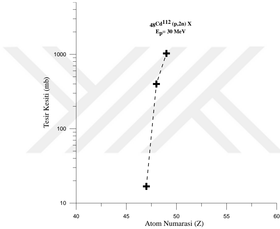
Şekil 4.23. Kadmiyum elementinin 30 MeV enerjili protonlarla bombardımanı sonucu oluşan ürün elementlerin oluşum tesir kesitleri
