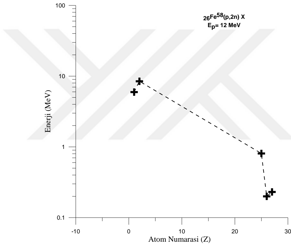
Şekil 4.33. Demir elementinin 12 MeV enerjili protonlarla bombardımanı sonucu oluşan ürün elementlerin enerji değerleri
