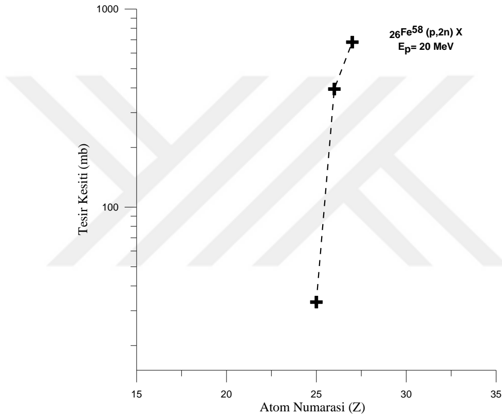
Şekil 4.39. Demir elementinin 20 MeV enerjili protonlarla bombardımanı sonucu oluşan ürün elementlerin oluşum tesir kesitleri
