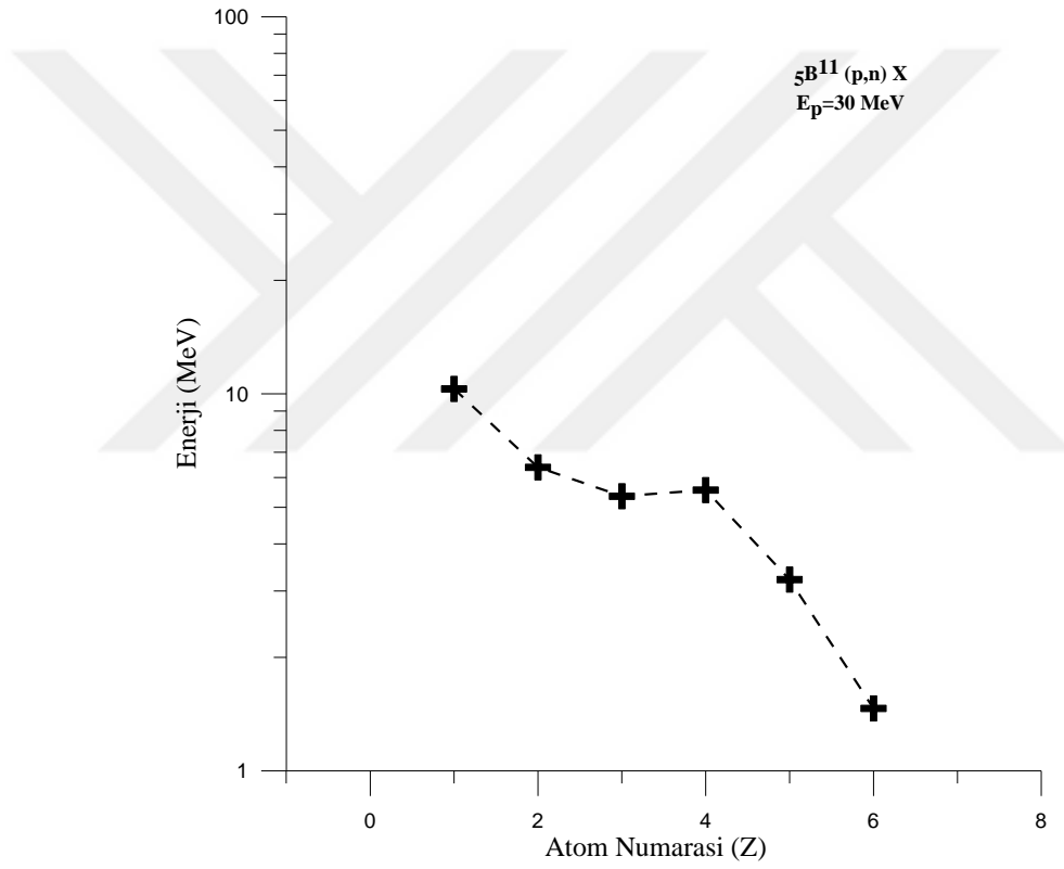
Şekil 4.6. Bor elementinin 30 MeV enerjili protonlarla bombardımanı sonucu oluşan ürün elementlerin enerji değerleri
