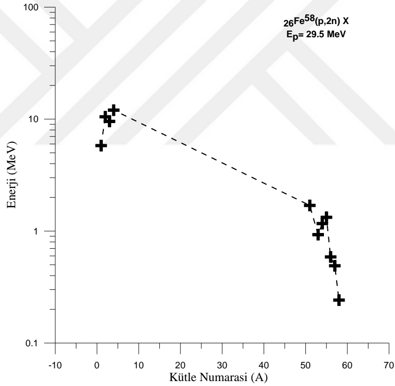
Şekil 4.45. Demir elementinin 29,5 MeV enerjili protonlarla bombardıman edilmesi sonucu oluşan ürün çekirdeklerin kütle dağılımı enerji değerleri
