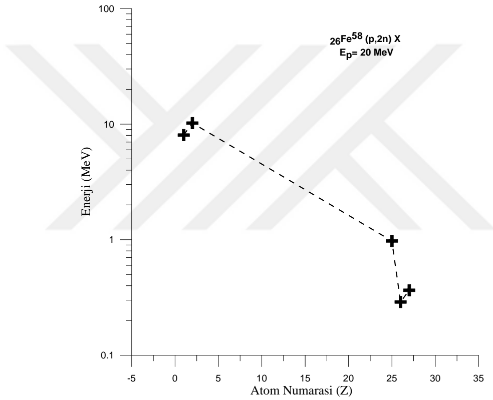
Şekil 4.38. Demir elementinin 20 MeV enerjili protonlarla bombardımanı sonucu oluşan ürün elementlerin enerji değerleri
