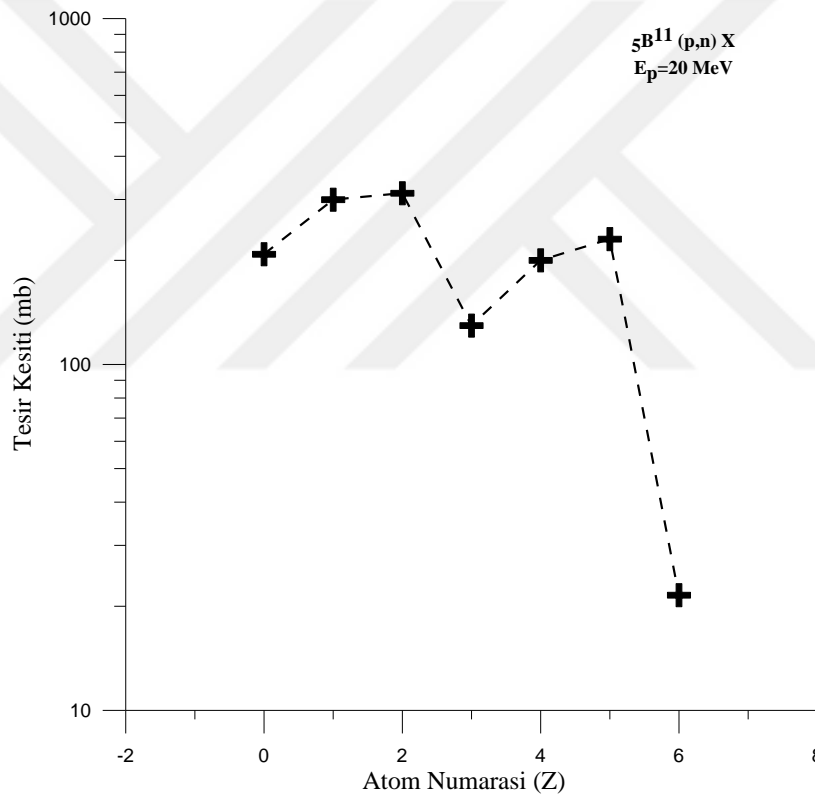
Şekil 4.2. Bor elementinin 20 MeV enerjili protonlarla bombardımanı sonucu oluşan ürün elementlerin oluşum tesir kesitleri
