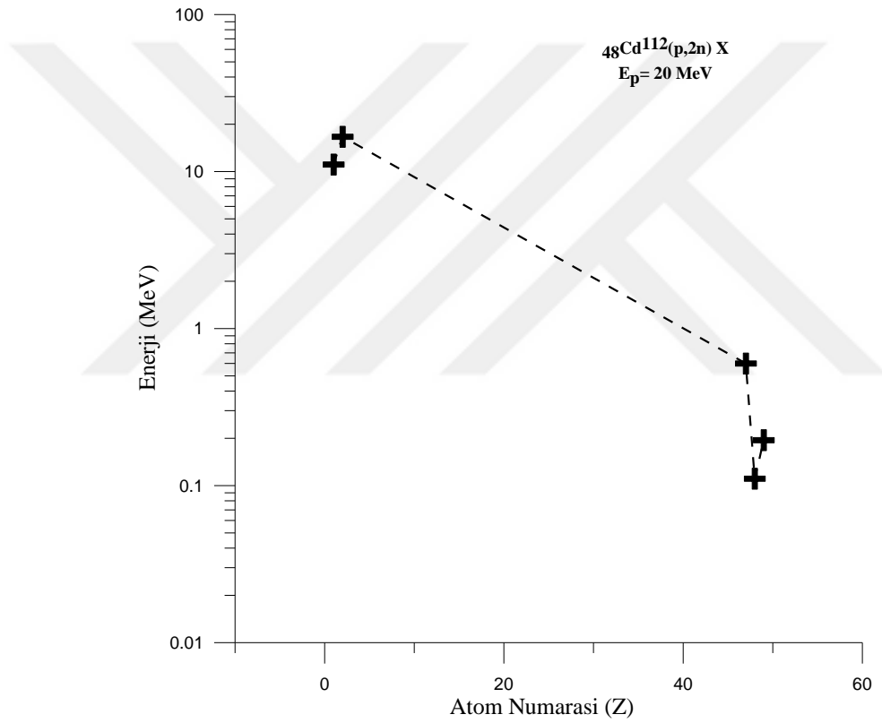
Şekil 4.17. Kadmiyum elementinin 20 MeV enerjili protonlarla bombardımanı sonucu oluşan ürün elementlerin enerji değerleri
