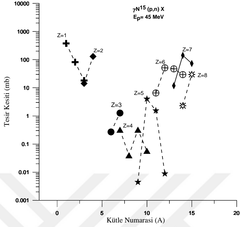
Şekil 4.63. Azot elementinin 45 MeV enerjili protonlarla bombardıman edilmesi sonucu oluşan ürün çekirdeklerin (Z=1-8) izotop üretim tesir kesiti değerleri
