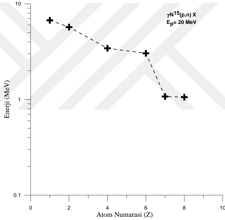
Şekil 4.49. Azot elementinin 20 MeV enerjili protonlarla bombardımanı sonucu oluşan ürün elementlerin enerji değerleri
