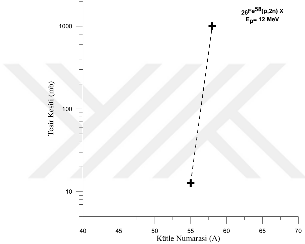
Şekil 4.36. Demir elementinin 12 MeV enerjili protonlarla bombardıman edilmesi sonucu oluşan ürün çekirdeklerin kütle dağılımı tesir kesiti değerleri
