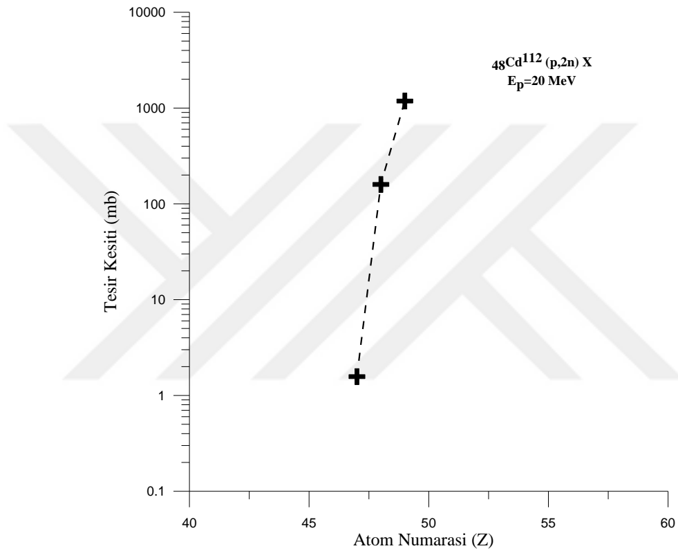
Şekil 4.18. Kadmiyum elementinin 20 MeV enerjili protonlarla bombardımanı sonucu oluşan ürün elementlerin oluşum tesir kesitleri
