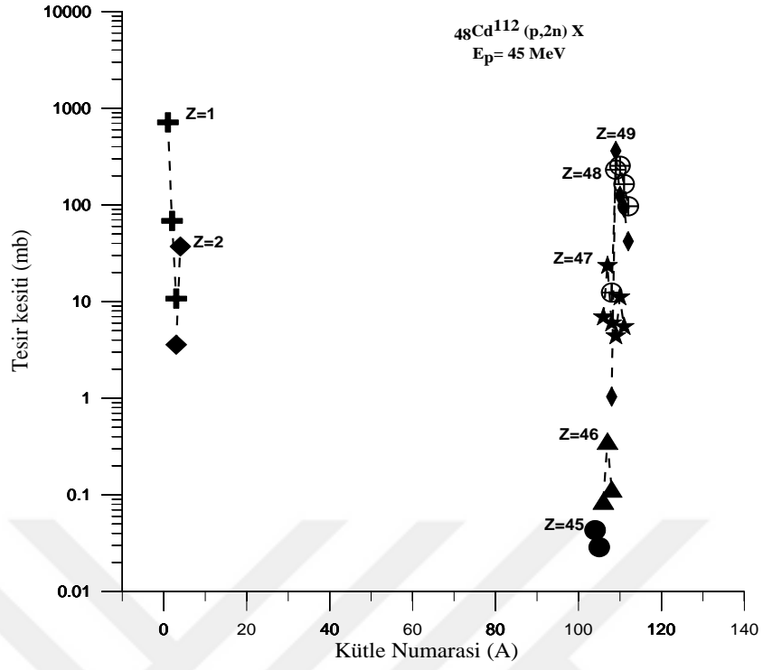
Şekil 4.31. Kadmiyum elementinin 45 MeV enerjili protonlarla bombardıman edilmesi sonucu oluşan ürün çekirdeklerin (Z=1,2,45,46,47,48,49) izotop üretim tesir kesiti değerleri
