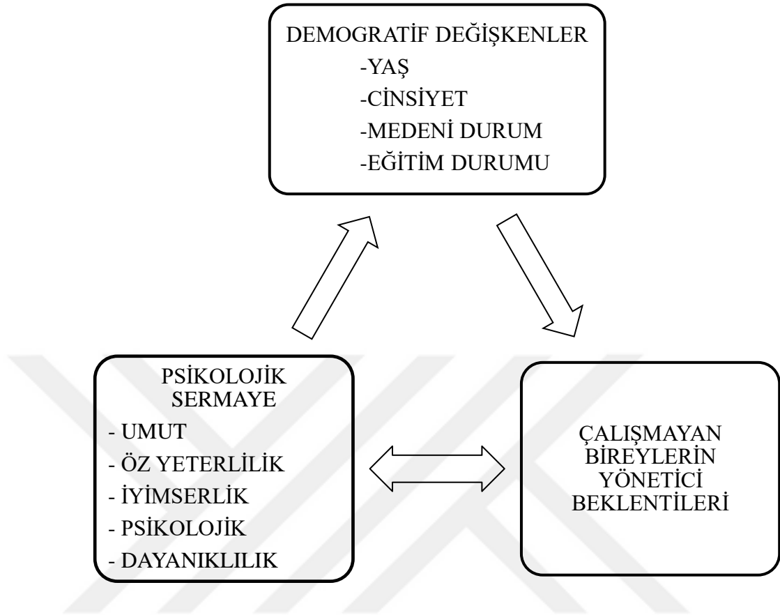
Şekil 4: Araştırma Modeli
