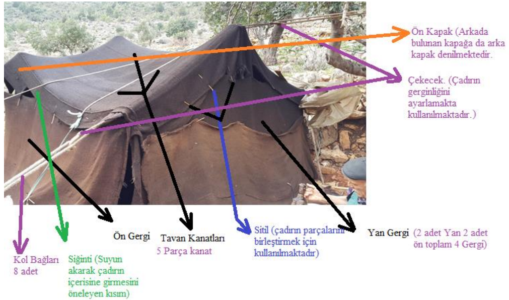
Şekil 11. Kurulmuş bir kara çadır görüntüsü ve parçaları
