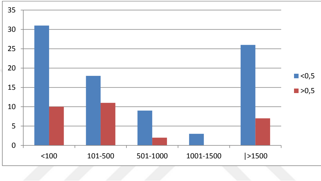
Şekil 4.13: Antikanser tedavi grubu PCT ile MNS arasındaki ilişki
