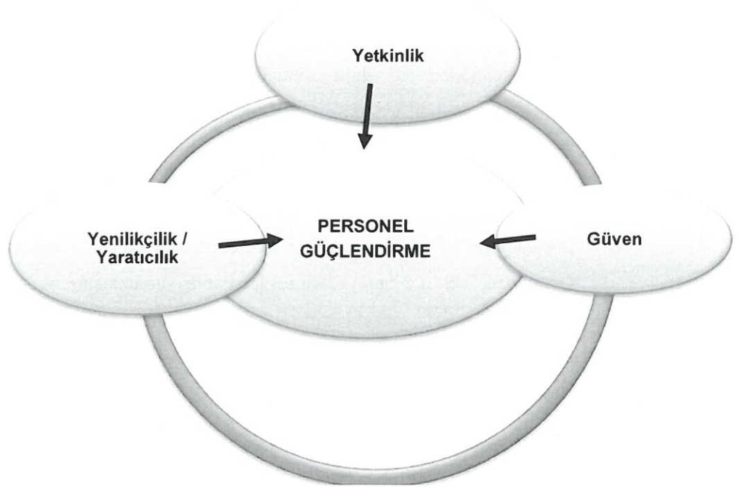
Şekil 1: Araştırma Analizi'nin Şematik Gösterimi
