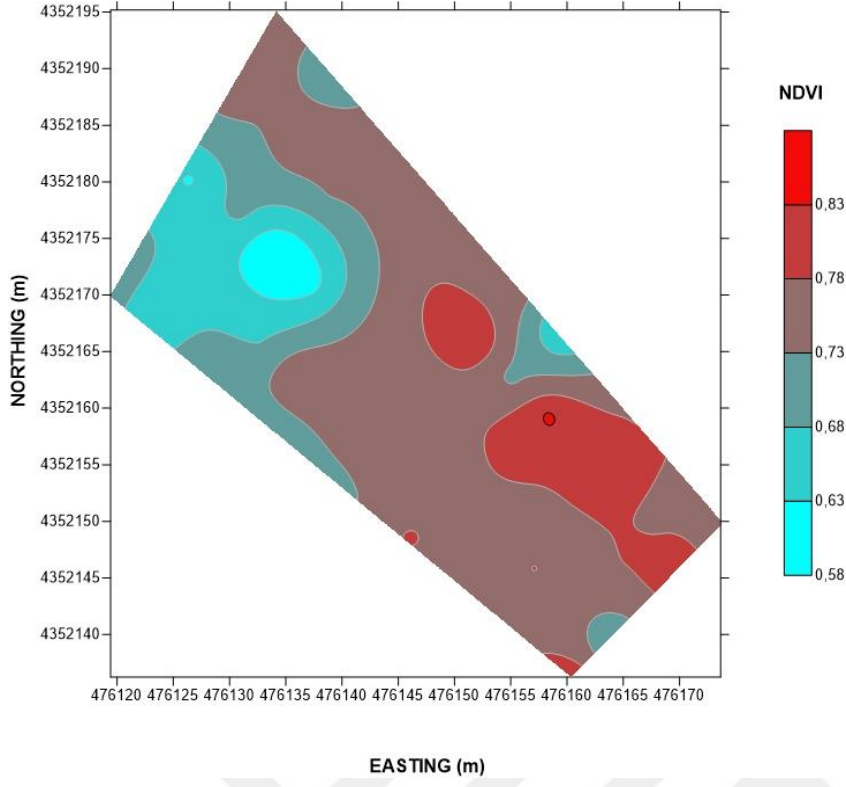
Şekil 4.7. Değişken düzeyli gübreleme yapılan ağaçlardan elde edilen NDVI haritası
