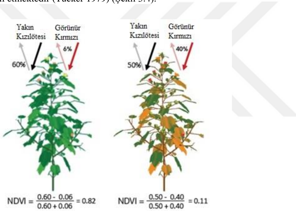
Şekil 3.4. Bitki sağlığına bağlı NDVI değerindeki değişim (GreenSeeker/Anonim, 2017)
