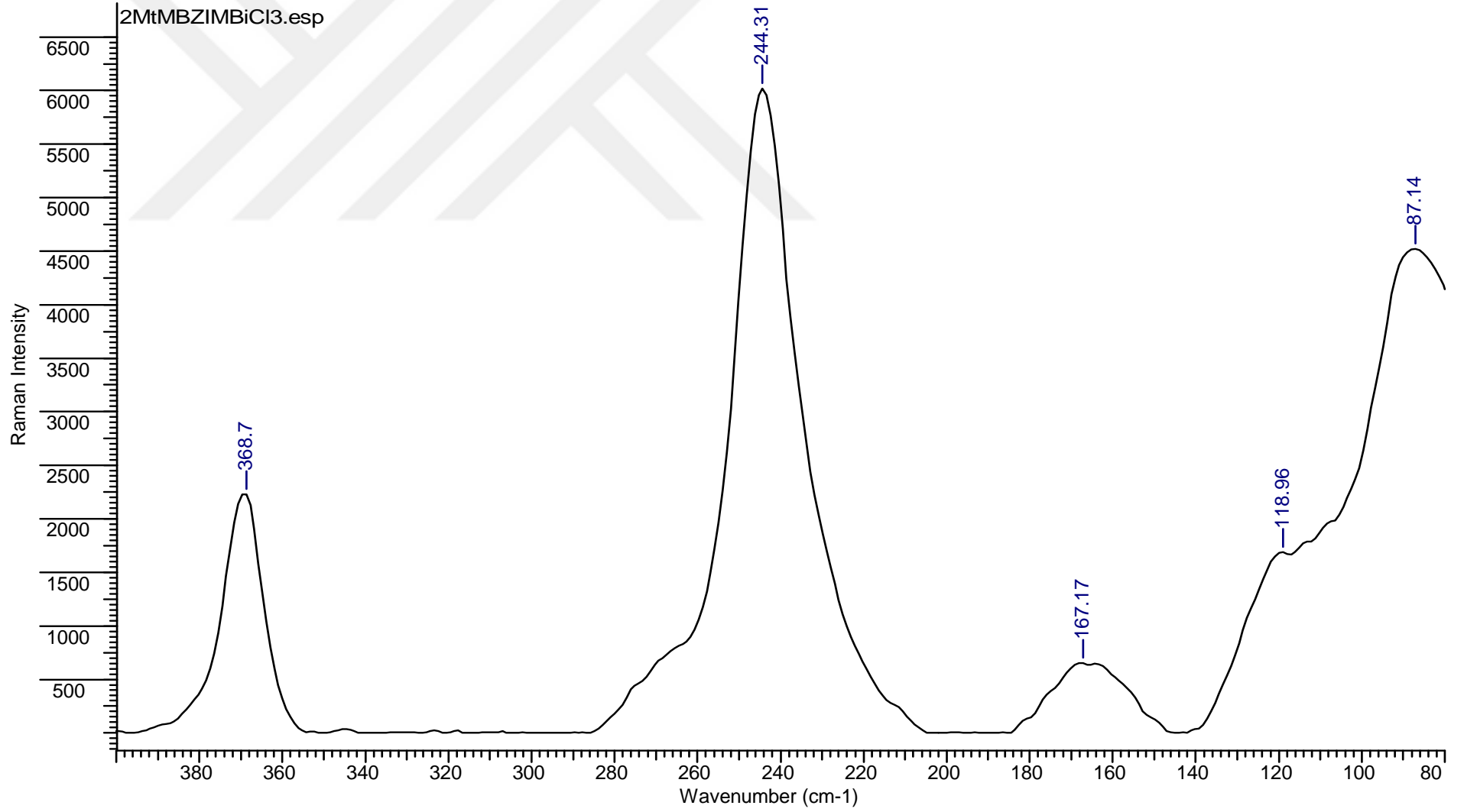
Şekil 7. 9 [\text{BiCl}_3(\text{MtMBZIM})_2 \cdot \text{aseton}] (2) bileşiğinin raman spektrumu
