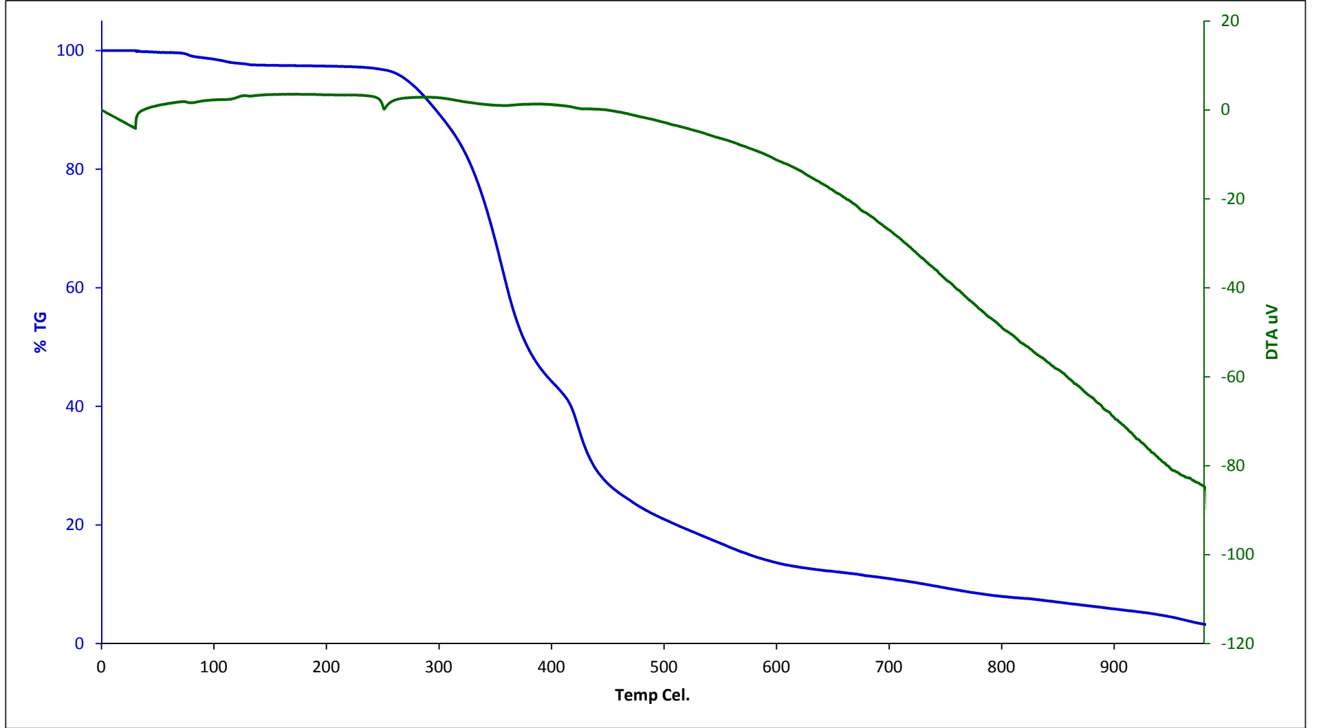
Şekil 7. 15 [\text{BiI}_3(\text{MtMBZIM})_2 \cdot \text{CH}_3\text{OH}]_2 (4) bileşiğinin TG-DTA eğrisi
