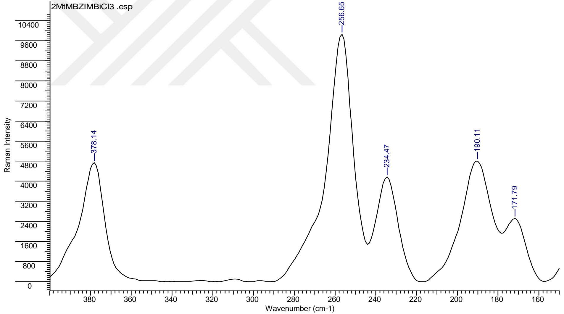
Şekil 7. 8 [\text{BiCl}_3(\text{MtMBZIM})_3 \cdot \text{aseton}] (1) bileşiğinin raman spektrumu
