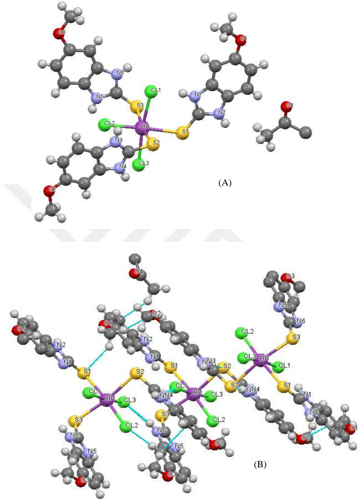
Şekil 7. 29 [\text{BiCl}_3(\text{MtMBZIM})_3 \cdot \text{aseton}] (1) bileşiğinin kristal yapısı (A) ve moleküler arası etkileşimler (B)
