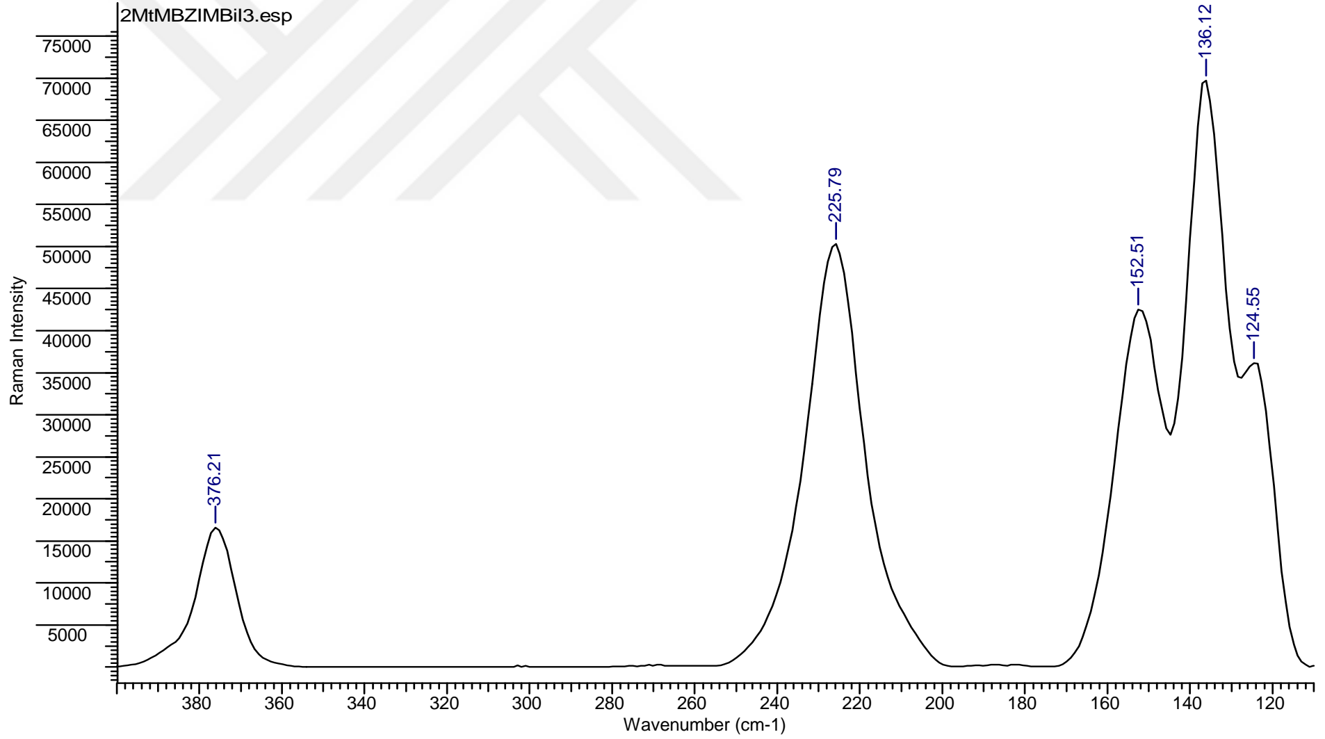
Şekil 7. 11 [\text{Bi}_3(\text{MtMBZIM})_2 \cdot \text{CH}_3\text{OH}]_2 (4) bileşiğinin raman spektrumu
