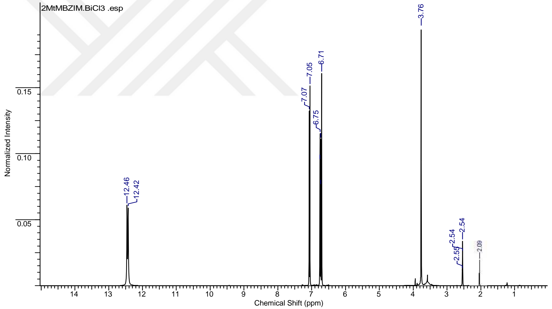
Şekil 7. 20 [BiCl 3 (MtMBZIM) 2 .aseton] (2) bileşiğinin 1 H NMR spektrumu
