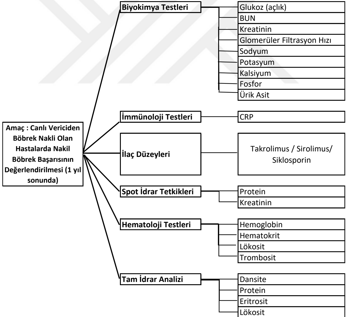
Şekil 5.1 Hiyerarşik Yapı
