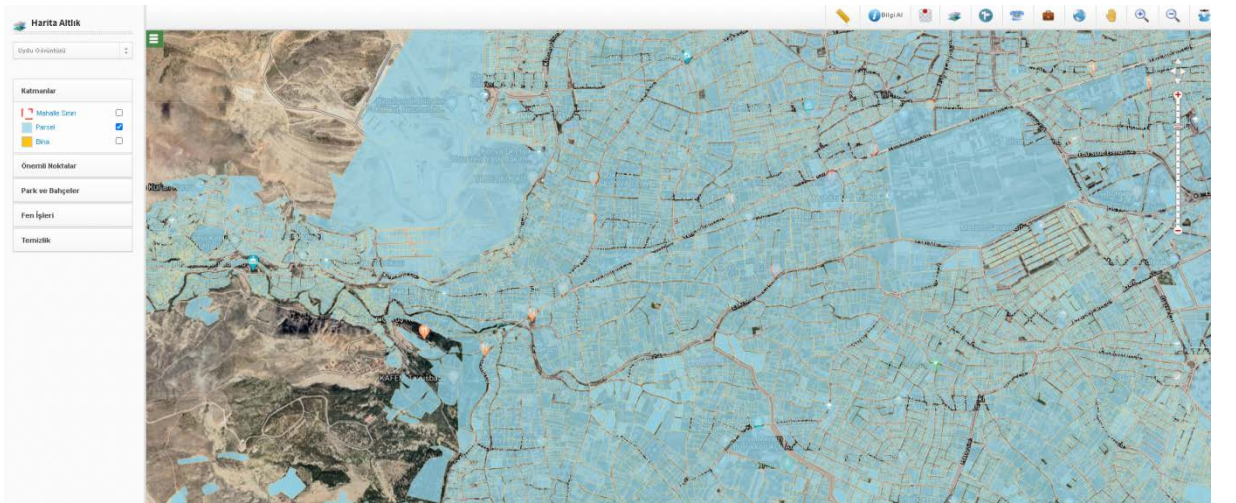
Şekil 42. Parsel katmanı
