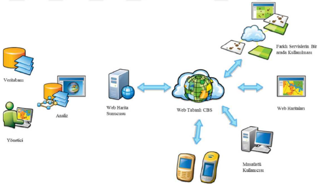
Şekil 3. Web cbs
