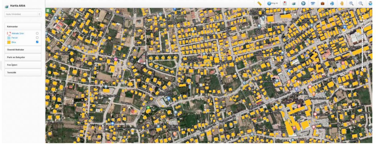
Şekil 43. Bina katmanı
