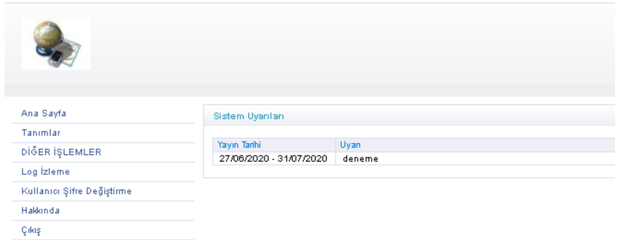
Şekil 79. Admin paneli
