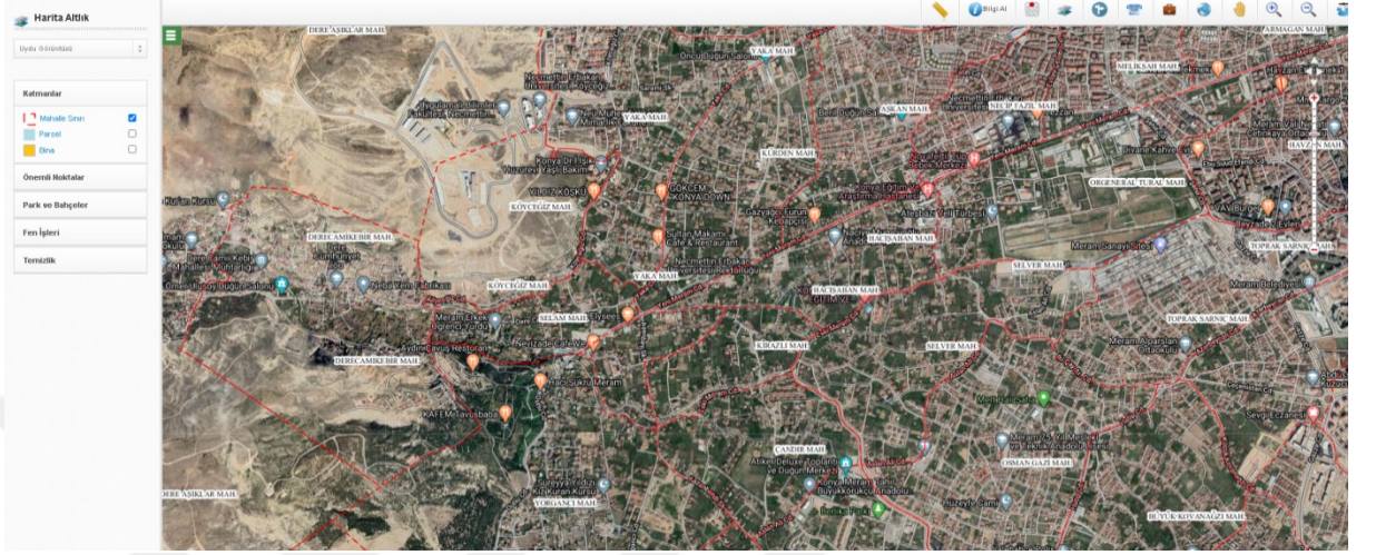
Şekil 41. Mahalle sınırları
