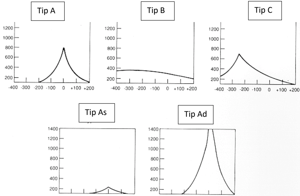
Şekil 2.3: Timpanogram çeşitleri (54)
