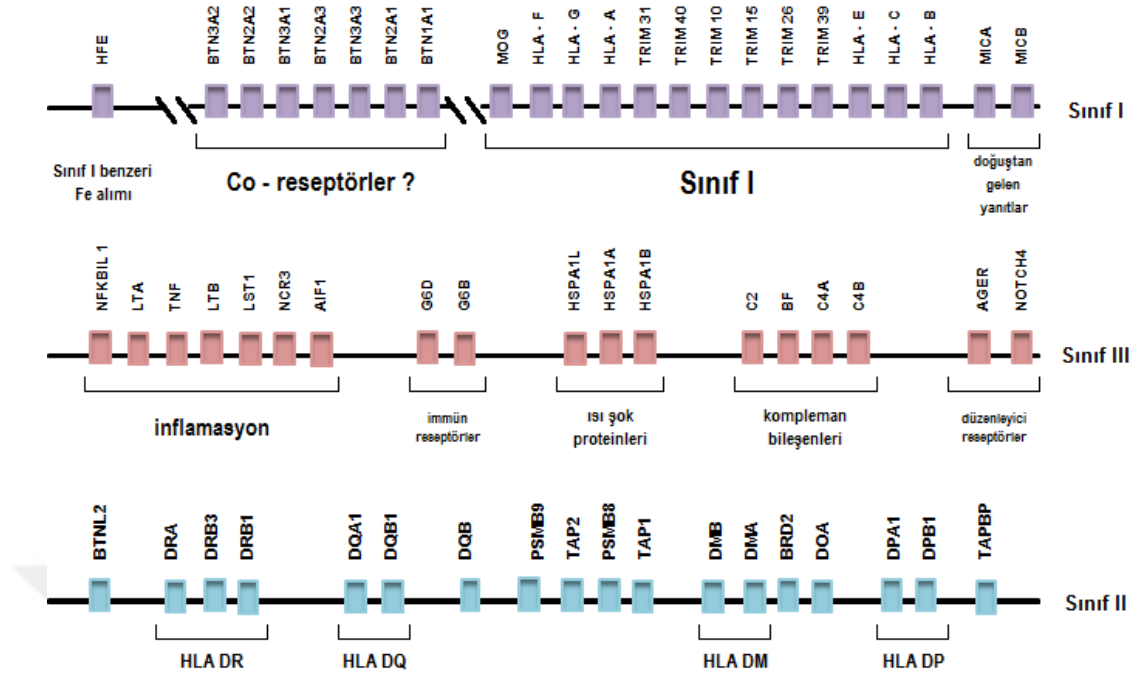
Şekil 2.1.: HLA'nın yapısı
