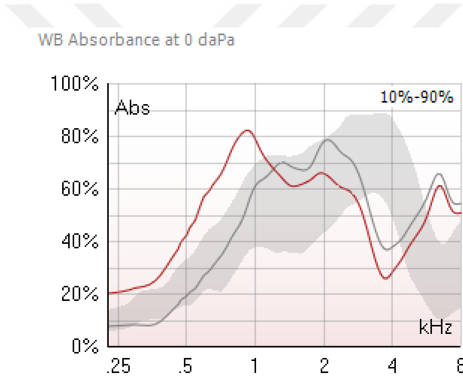
Resim 8. Absorbans Grafiği
