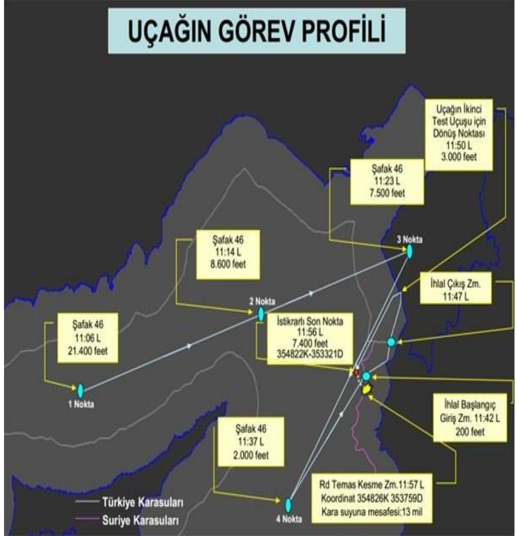
- Şekil-7- ( Türk Jetinin Radar İzi)
