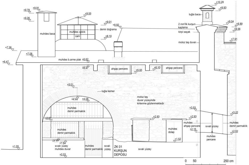
Şekil 2.28. Z01 mekanı, B-B kesiti (Tures Turizm Planlama ve Restorasyon San. ve Tic. Ltd. Şti., 2009)
