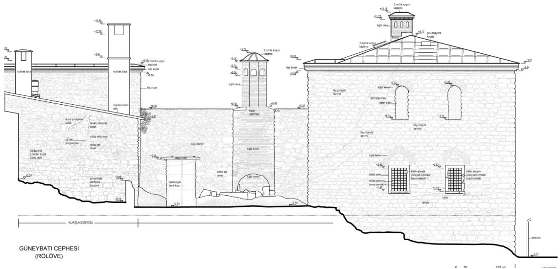
Şekil 2.24. Erzak Kapısı ve Mutfaklar bölümünü de gösteren güneybatı görünüşü (Tures Turizm Planlama ve Restorasyon San. ve Tic. Ltd. Şti., 2009)
