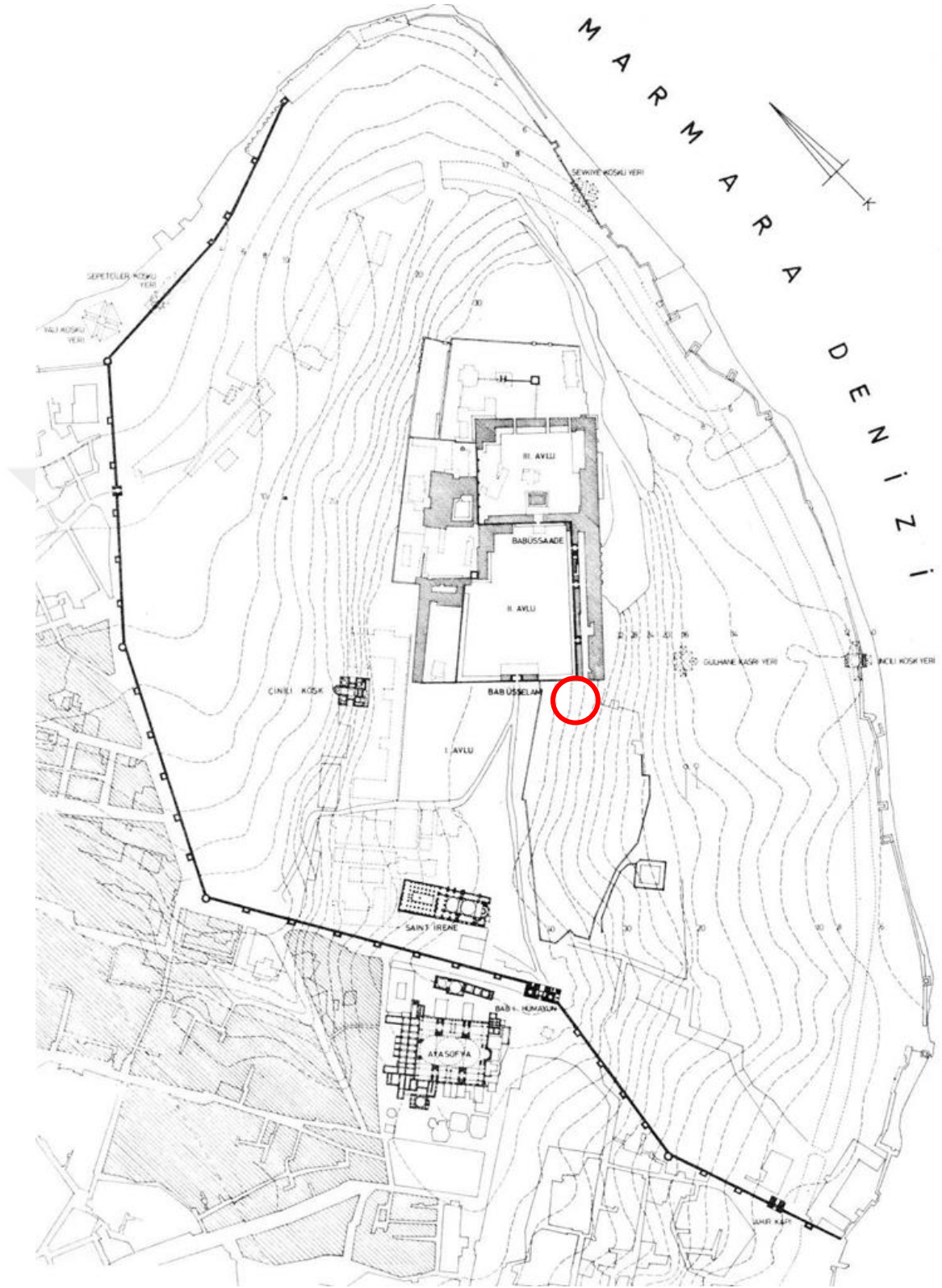
Şekil 2.10. 1871–73 döneminden demiryolunun geçirilmesine kadar Sur-u Sultani'nin görünüşü (Eldem & Akozan, 1982)
