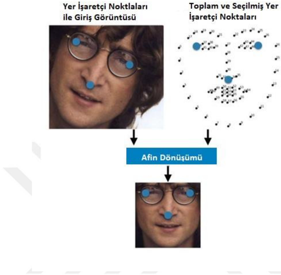
Şekil 4. 5. Görüntüdeki yüze afin dönüşümü işleminin uygulanma görseli. (Amos, Ludwiczuk ve Satyanarayanan, 2016).
