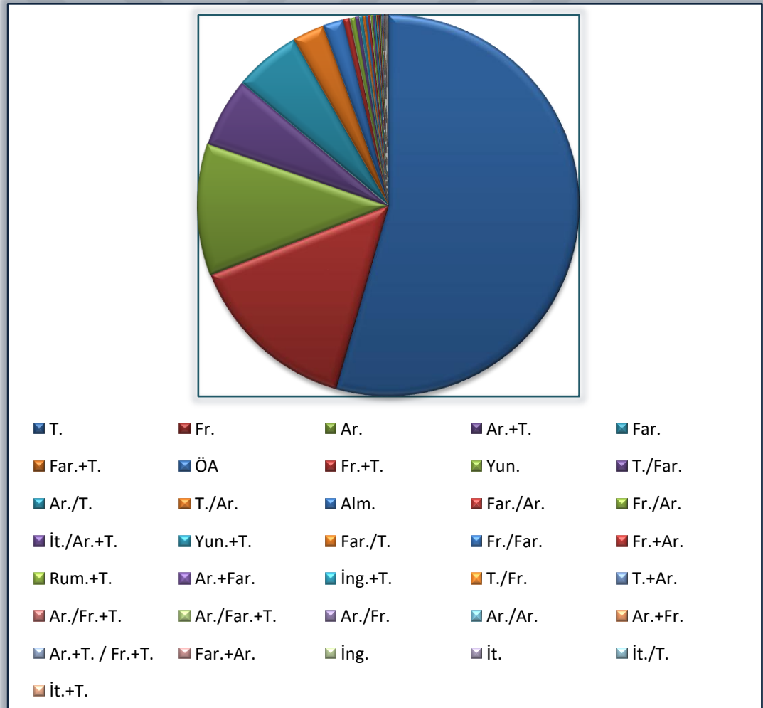
Şekil 3.4. Kaynak Dillerine Göre Niteleme Sıfatları Grafiği
