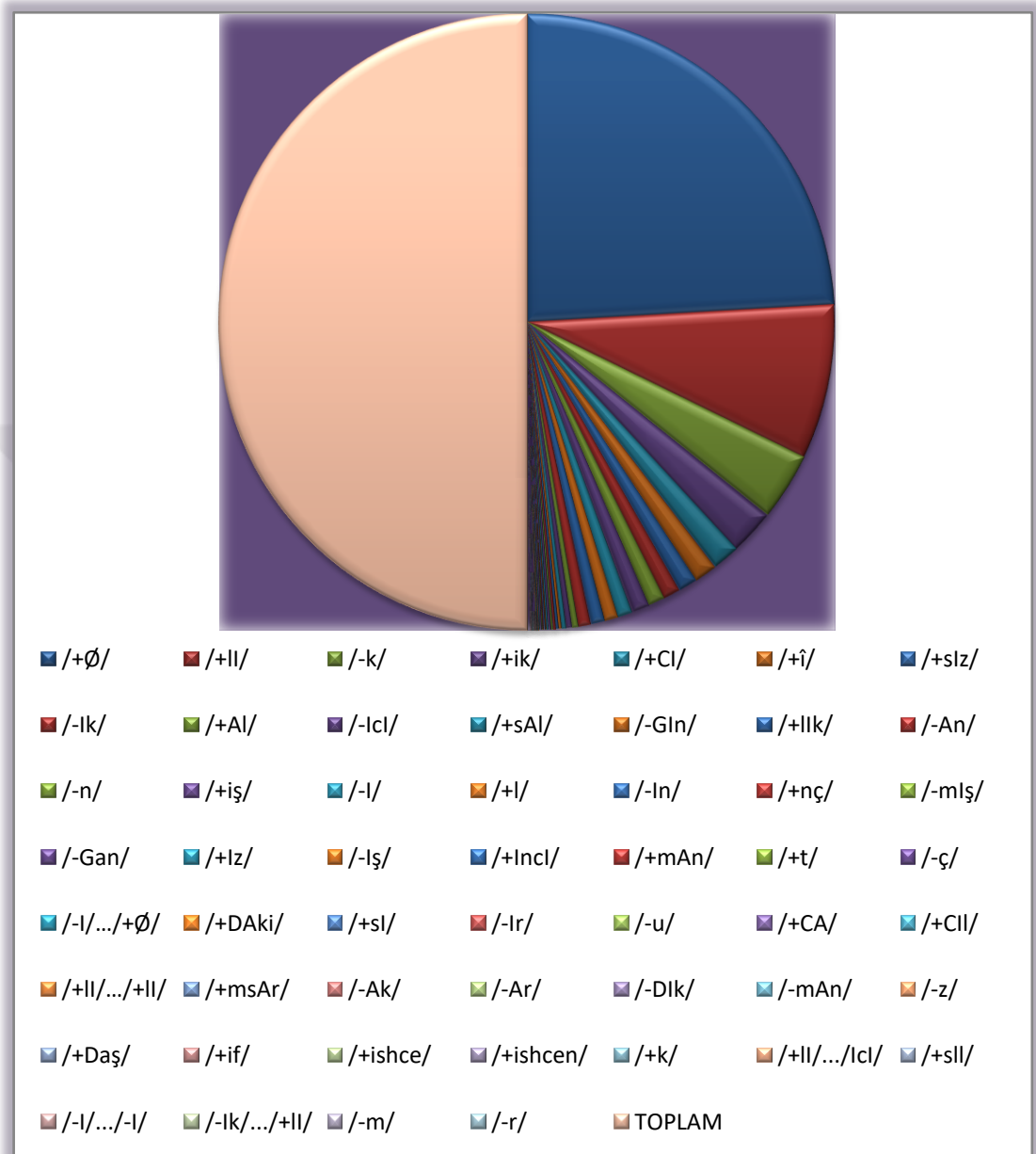
Şekil 3.3.1.Sözcük Halindeki Niteleme Sıfatı Grafiği
