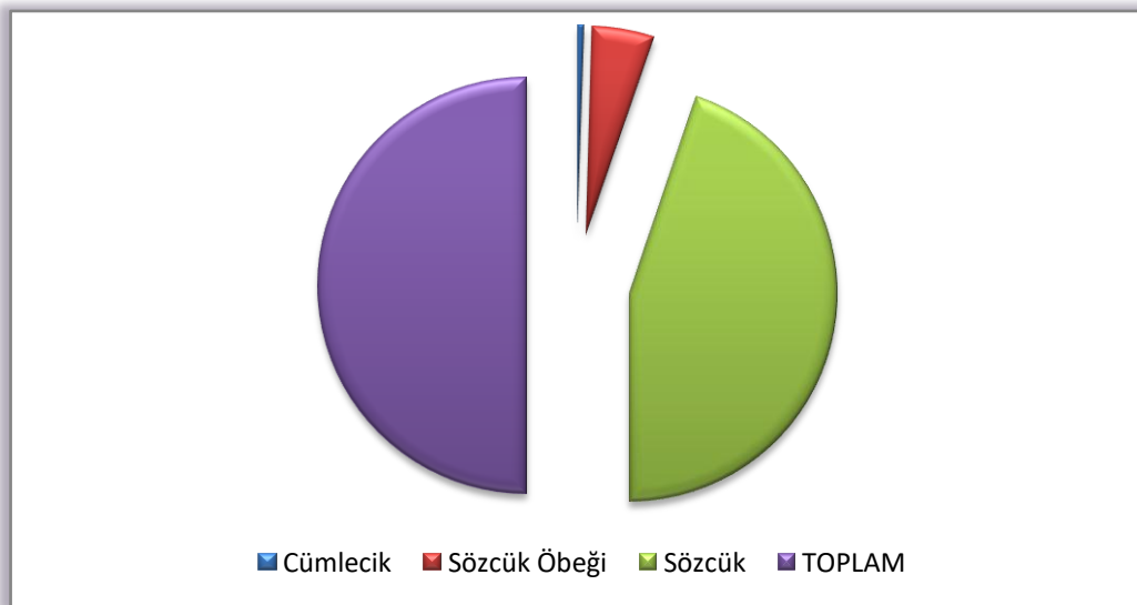
Şekil 3.3. Yapılarına Göre Niteleme Sıfatları Grafiği
