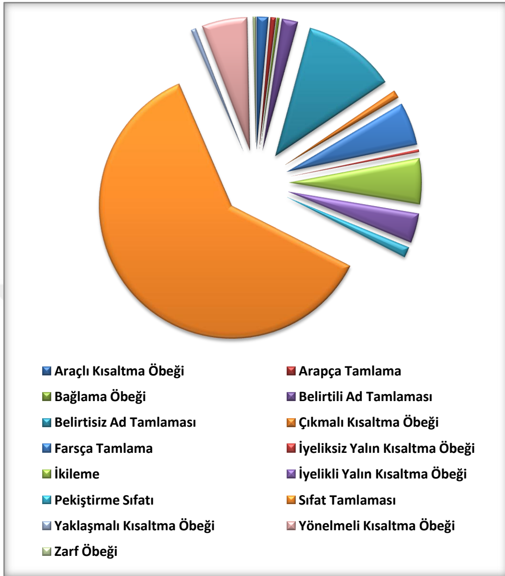
Şekil 3.3.2. Sözcük Öbeği Halindeki Niteleme Sıfatları Grafiği
