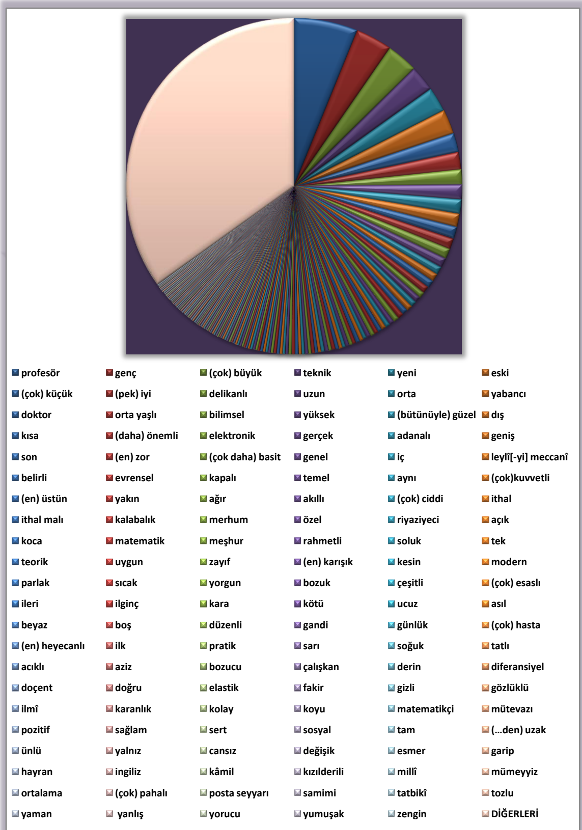
Şekil 3.2. Niteleme Sıfatları Geçiş Sıklığı Grafiği
