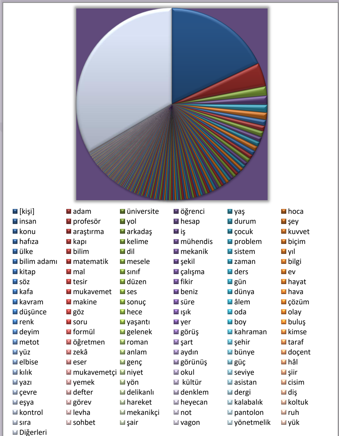
Şekil 3.5. Birlikte Kullanıldıkları Adlara Göre Niteleme Sıfatları Grafiği
