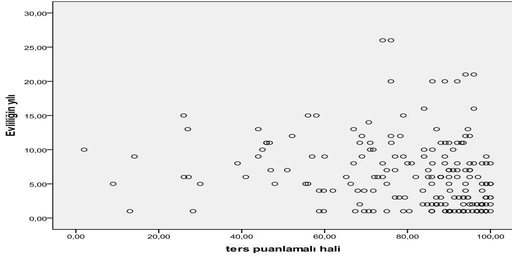
Şekil 4.7: Saçılım Grafiği
