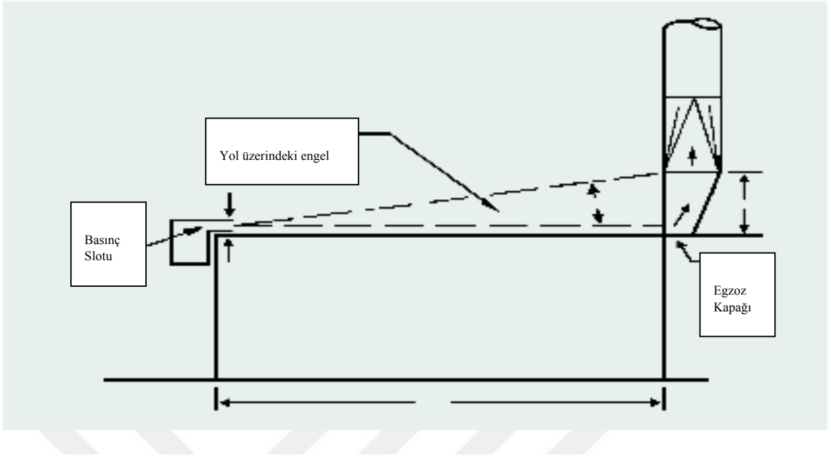
Şekil 5.3: İtme çekme davlumbazı [17]
