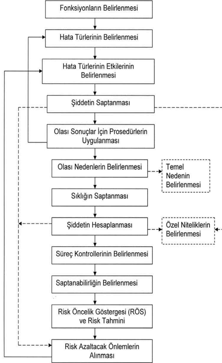
Şekil 3.5: FMEA prosesi [9]
