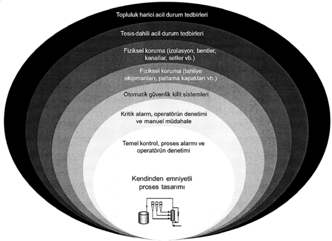
Şekil 3.8: LOPA katmanları [9]
