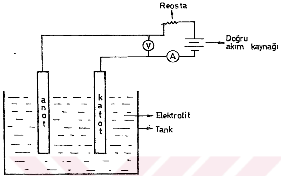
Şekil 4.1: Elektrometal Kaplama Prosesi[15]
