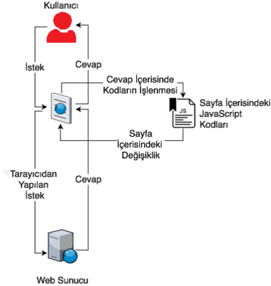
Şekil 3.10 : DOM tabanlı XSS zafiyeti
