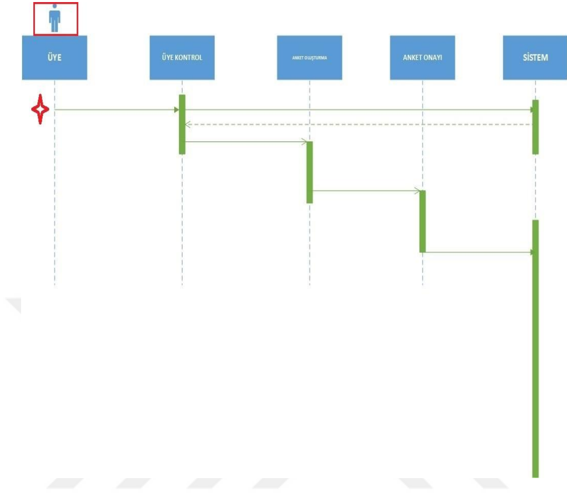
Şekil 3.12 : Yazılım tasarımı örneği
