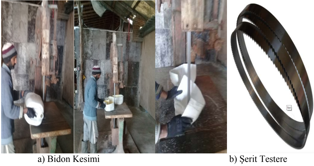
Şekil 2.34: Şerit Testere Kesim Makinesi
