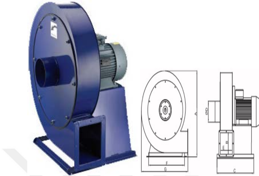
Şekil 2.37: Taşıyıcı fan kısımları
