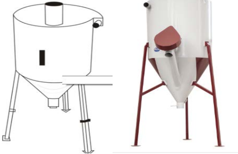
Şekil 2.38: Paketleme silosu makinesinin
