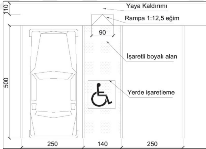
Şekil 2.18 Açık otopark park planı ve kullanılan işaretler (TS 12576, 2012)
