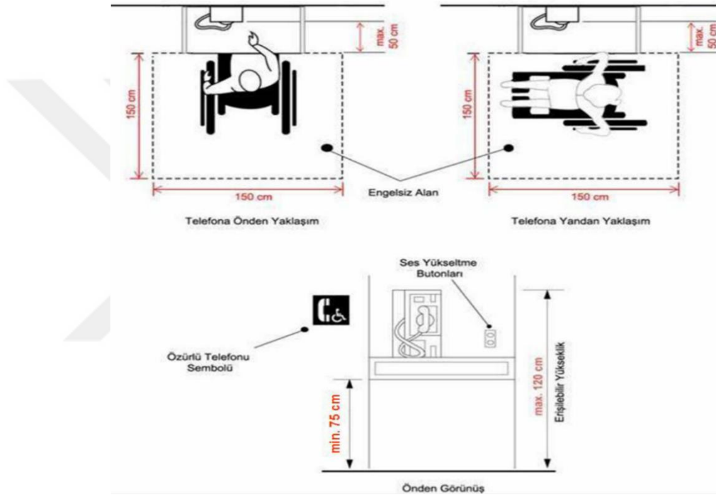
Şekil 2.38 Telefon kulübesi boyutları (T.C. Aile ve Sosyal Politikalar Bakanlığı Özürlü ve Yaşlı Hizmetleri Genel Müdürlüğü, 2011)
