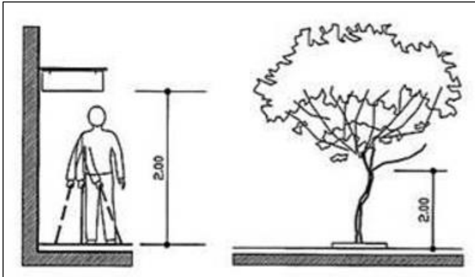
Şekil 2.9 Sarkan dal, tabela ve levha yükseklikleri (ÖZİDA, 2010)
