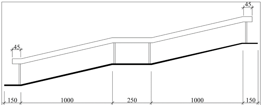
Şekil 2.10 Eğim ve sahanlık alanları (ÖZİDA, 2010)
