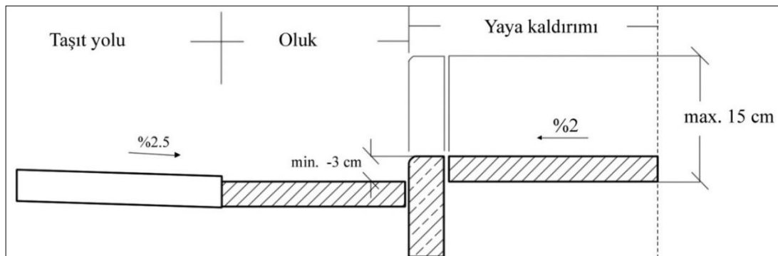
Şekil 2.7 Bordür taş yüksekliği (ÖZİDA, 2010)
