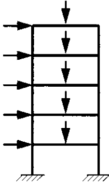
Şekil 2.6: Yapının Davranışı
