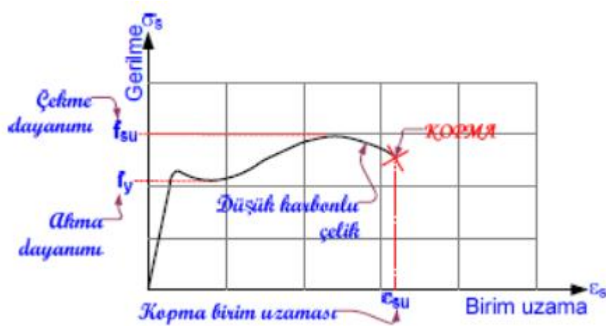
Şekil 2.1: Çelik Çekme Grafiği
