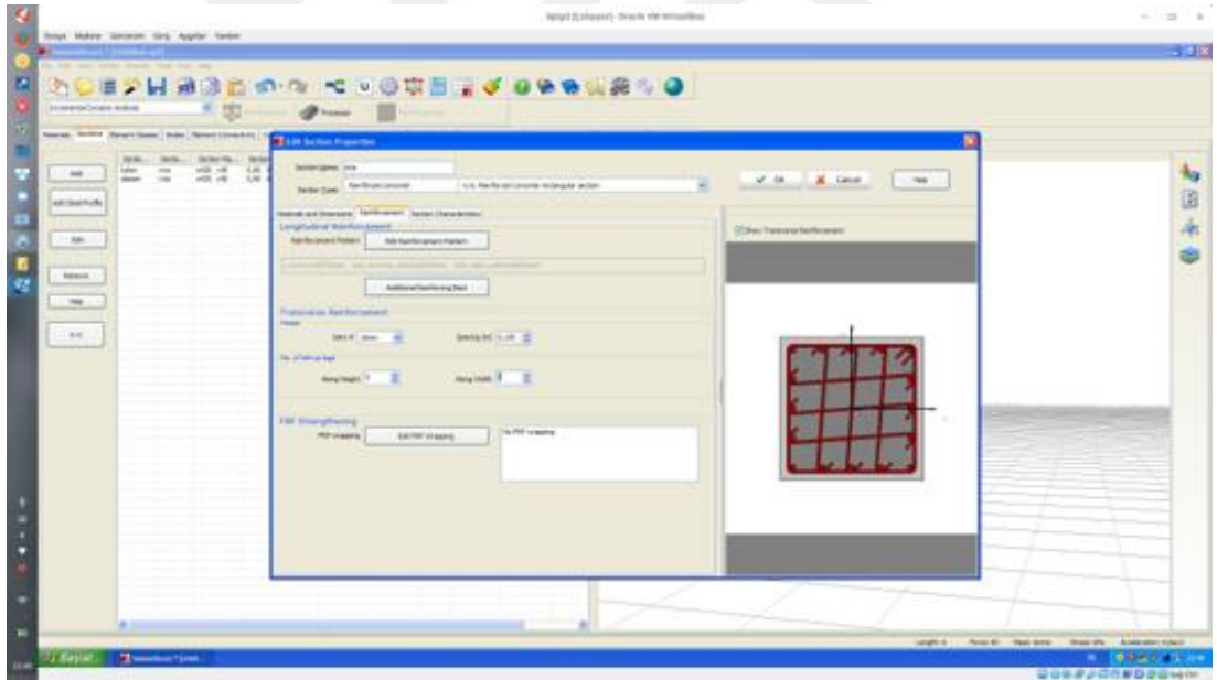
Şekil 3.5: Seismo Struct programından 6 katlı tasarımın yapının donatı kesiti Betonarme yapının donatı dizilişinin ve kullanılan malzeme içeriği görünmektedir.
