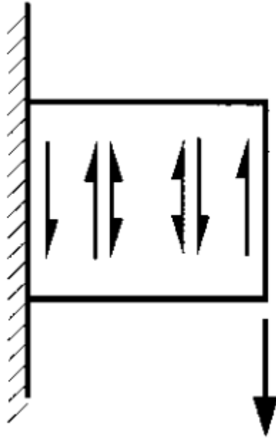
Şekil 2.4: Yapının Davranışı
