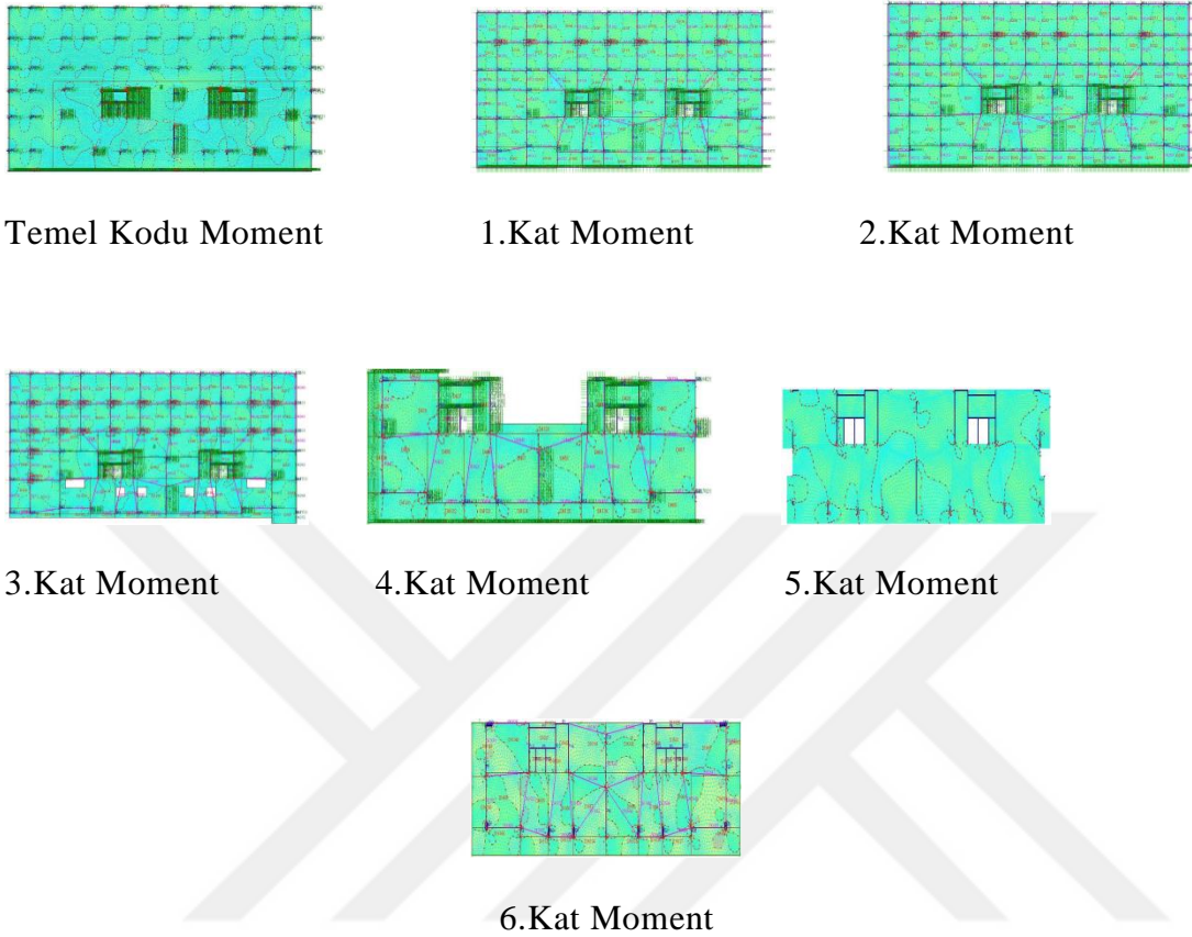
Şekil 3.16: ProBina Yapı kodlarının moment x-y göstergeleri
