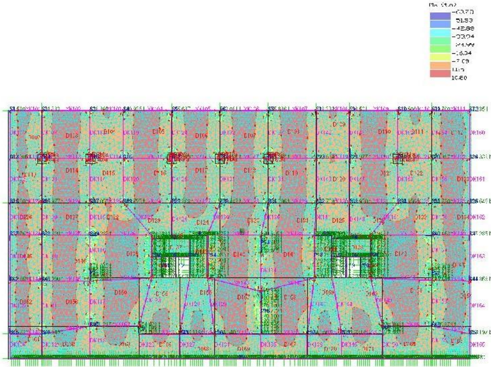
Şekil 3.13: ProBina 1.Kat kodu moment-x yönü dayanımı
