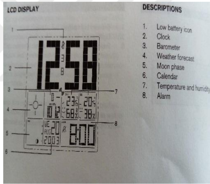
Şekil 24 Çok fonksiyonel termometre(higrometre ve barometre)
