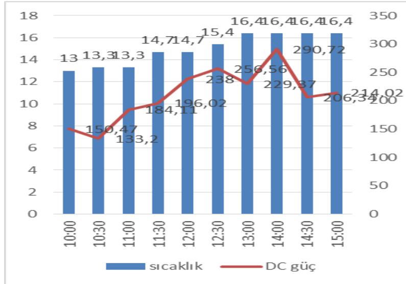
Şekil 31 Sıcaklık-DC Güç Değişimi-15/12/2017
