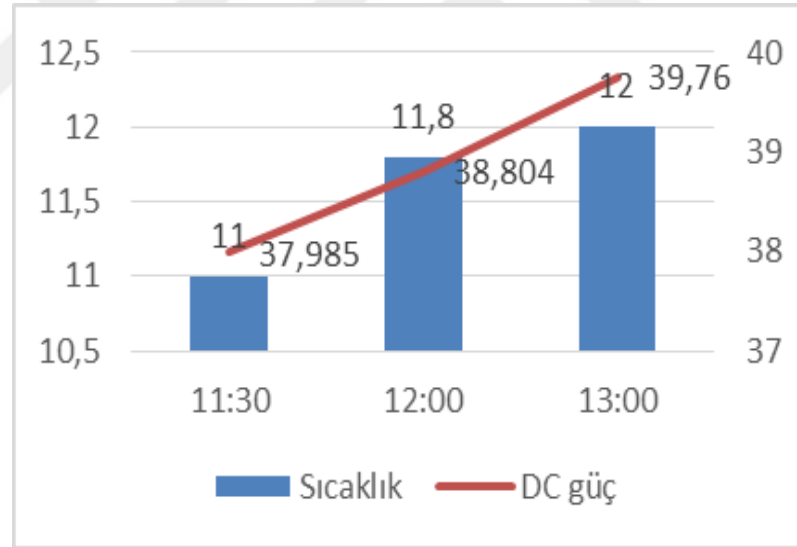
Şekil 27 Sıcaklık-DC Güç Değişimi-27/11/2017
