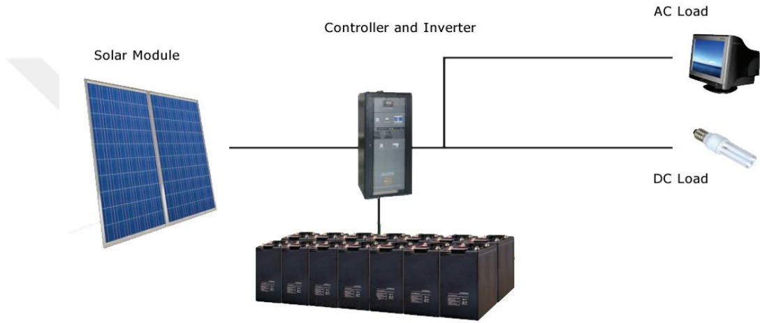
Şekil 2 Off-grid Güneş Enerjisi Sistemi
