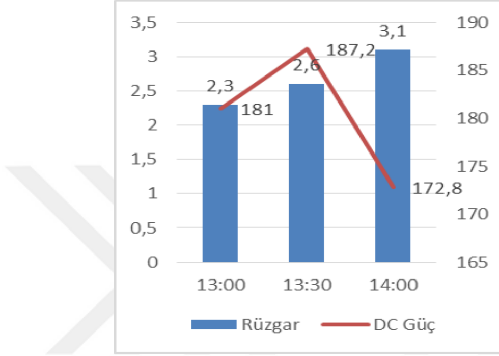
Şekil 43 Rüzgar-DC Güç Değişimi-07\12\2017
