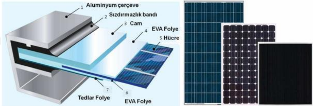
Şekil 3.3 Fotovoltaik Panel Kesiti
