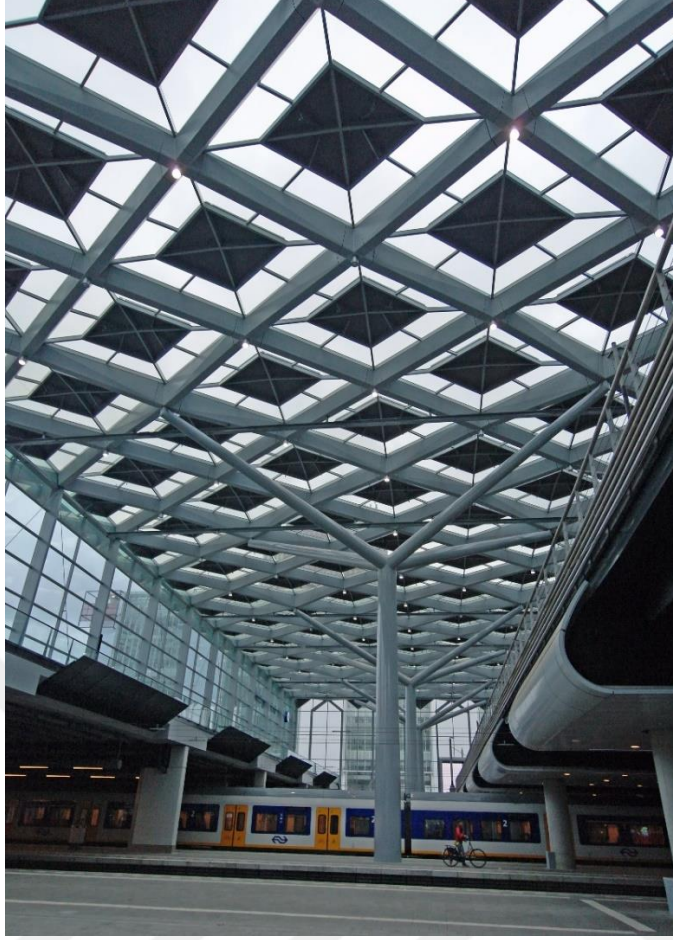
Şekil 2.25 Hollanda Tren İstasyonunda Çatıda Kullanılan Fotovoltaik Paneller
