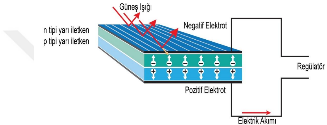
Şekil 3.2 Fotovoltaik Hücrenin Enine Kesiti
