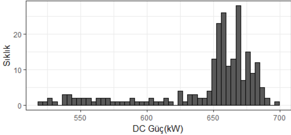
Şekil 29. 21 Aralık 2015 DC Güç Sıklık Dağılımı
