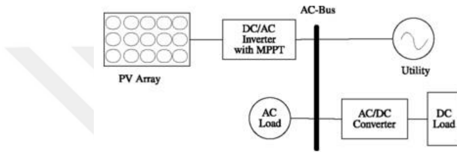
Şekil 4. Şebekeye bağlı PV sisteminin topolojisi
