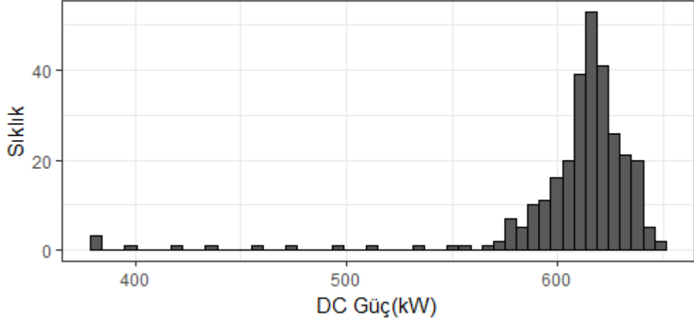
Şekil 45. 4 Temmuz 2015 DC Güç Sıklık Dağılımı
