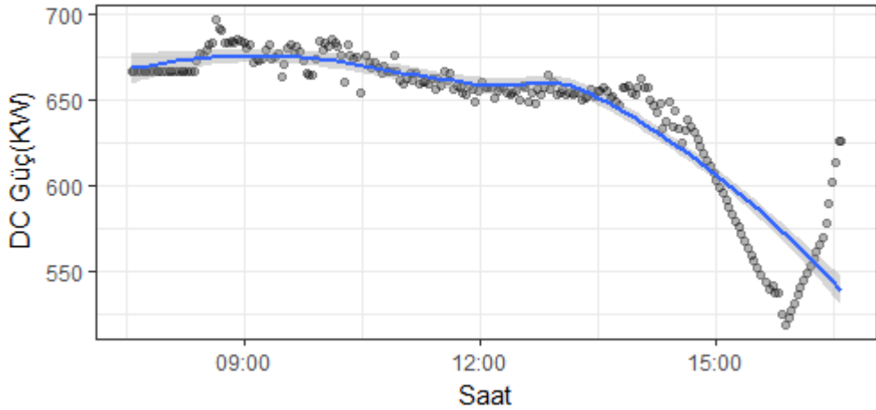
Şekil 30. 21 Aralık 2015 DC Güç Zaman
