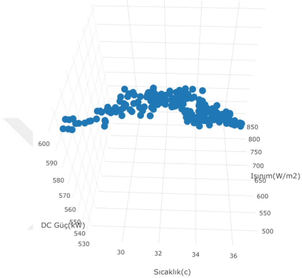
Şekil 27. 21 Haziran 2015 Sıcaklık Işınım DC Güç Değişim Grafiği
