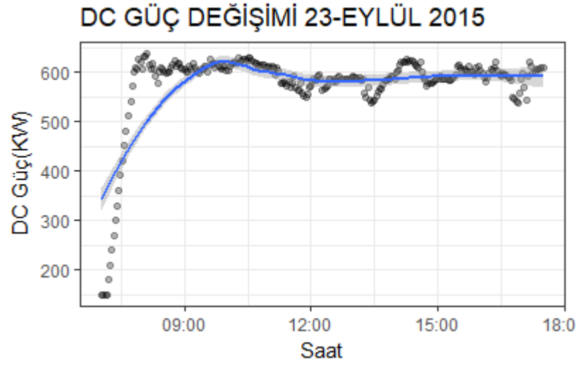
Şekil 14. 23 Eylül 2015 DC Güç Zaman
