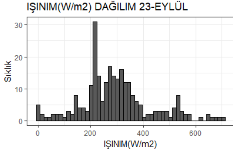
Şekil 17. 23 Eylül 2015 İşinim Sıklık Grafiği
