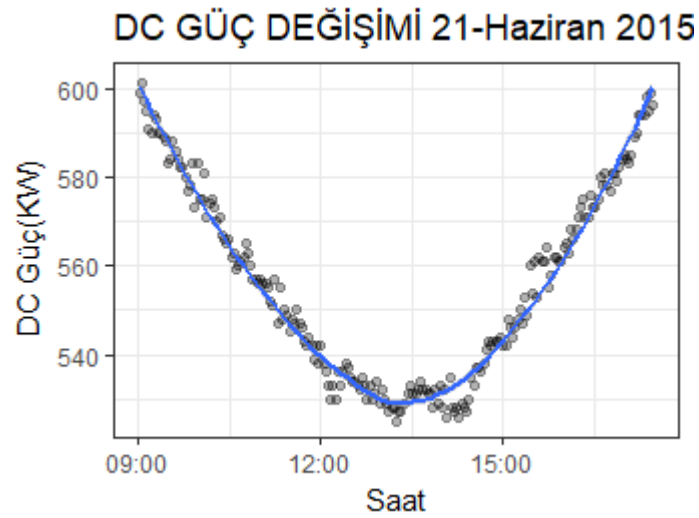
Şekil 22. 21 Haziran 2015 DC Güç Zaman
