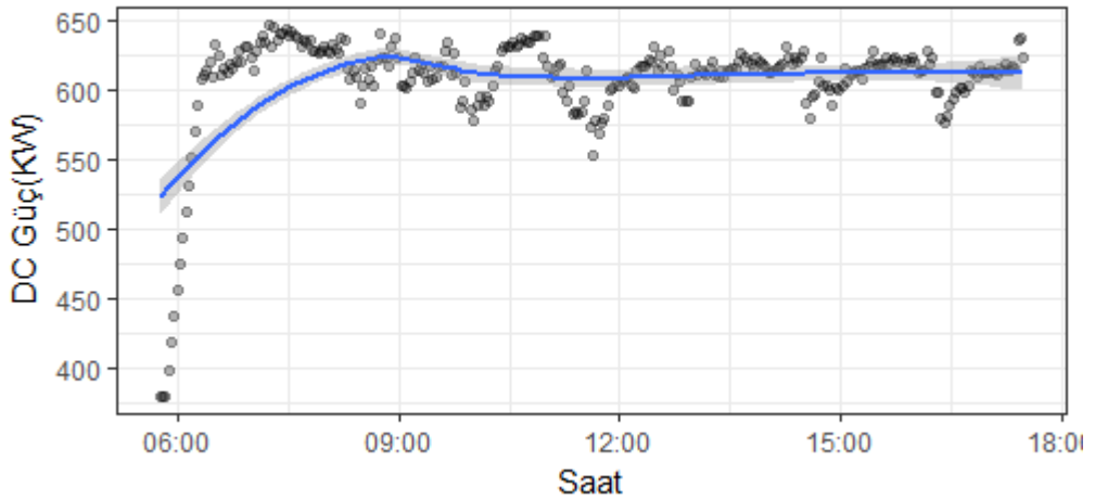
Şekil 46. 4 Temmuz 2015 DC Güç Zaman
