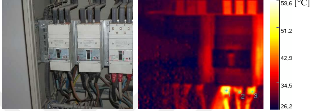
Resim 4.30. Standart ve kızılötesi termal kamera fotoğrafları 29
