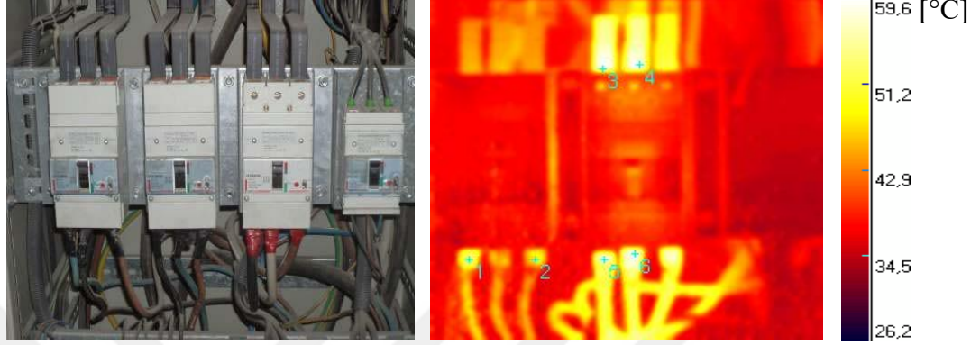
Resim 4.31. Standart ve kızılötesi termal kamera fotoğrafları 30
