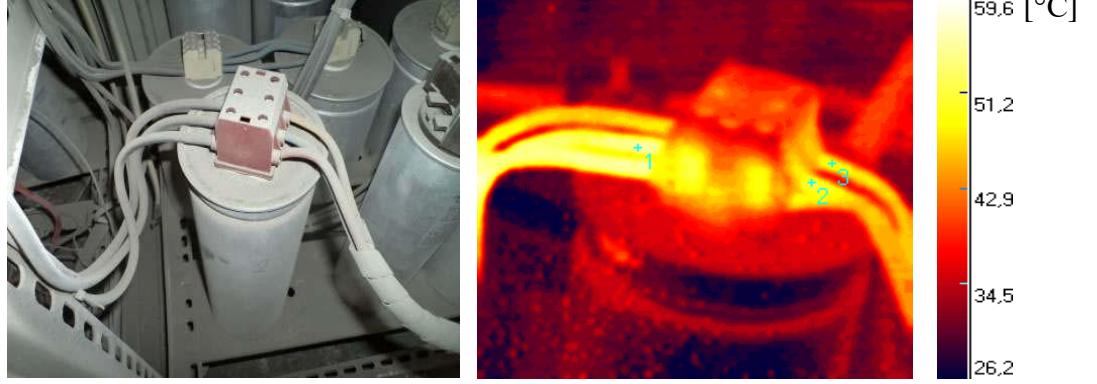
Resim 4.18. Standart ve kızılötesi termal kamera fotoğrafları 17
