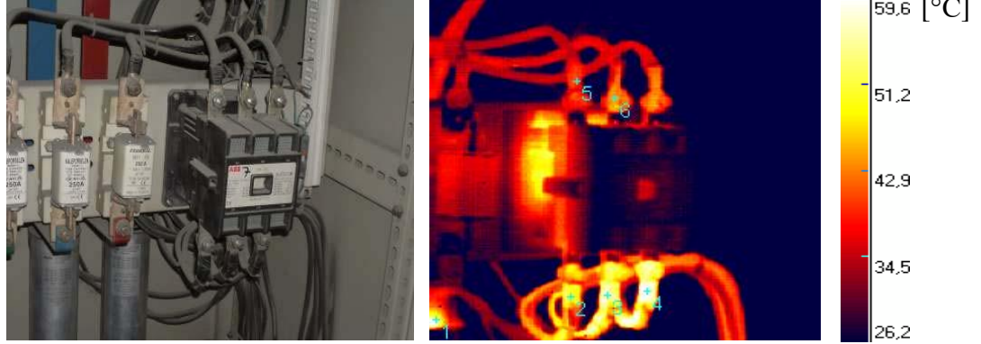
Resim 4.7. Standart ve kızılötesi termal kamera fotoğrafları 6
