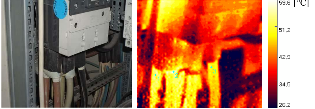
Resim 4.25. Standart ve kızılötesi termal kamera fotoğrafları 24
