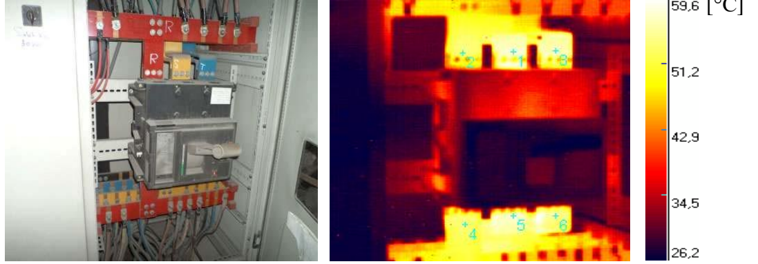
Resim 4.9. Standart ve kızılötesi termal kamera fotoğrafları 8
