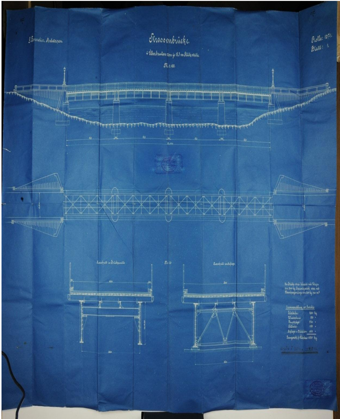
Ek 12: Yeşilirmak üzerine yapılması planlanan köprünün projesi
