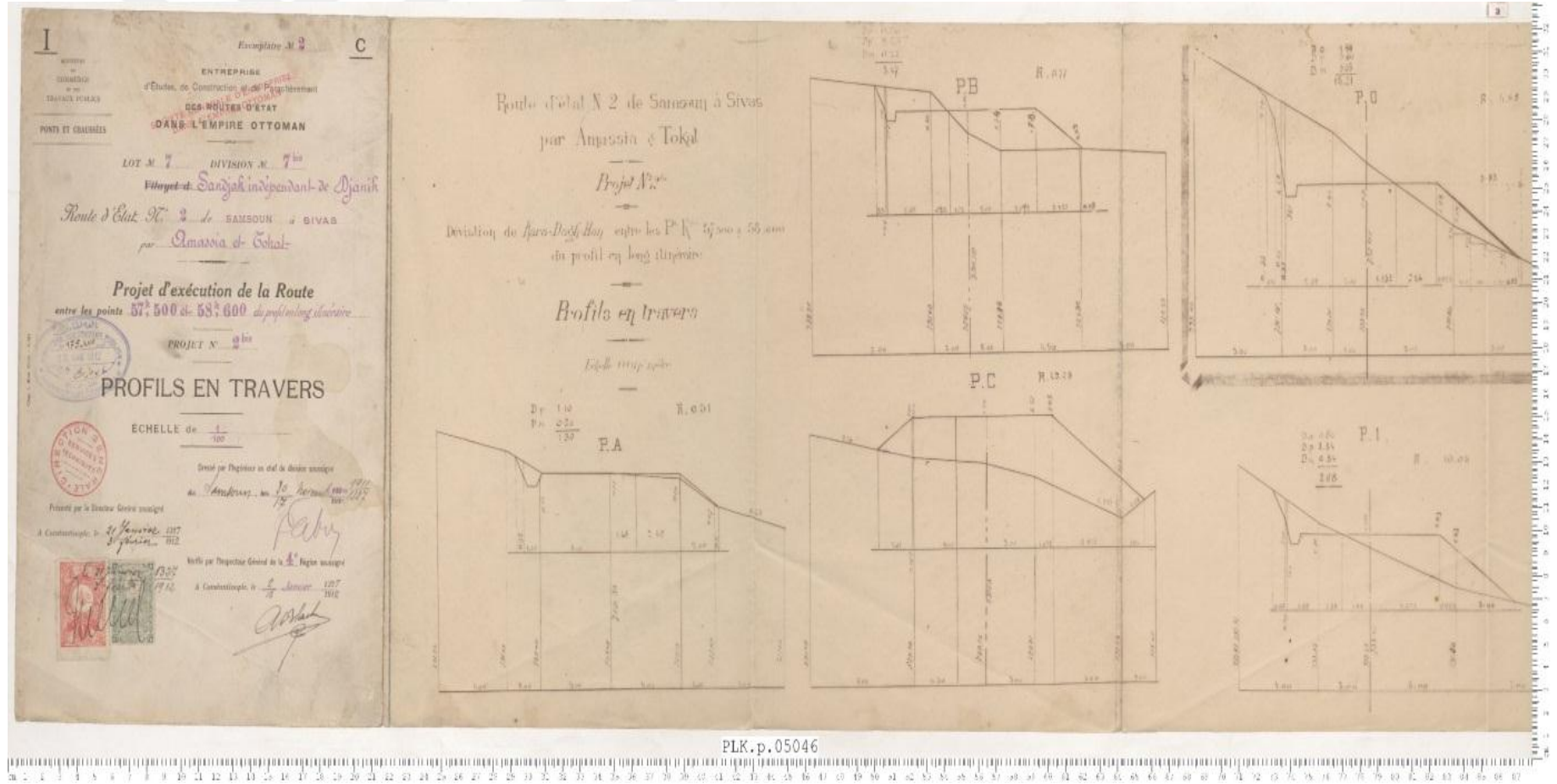
Resim 9: Samsun-Sivas, Amasya-Tokat demiryolu travers planı
