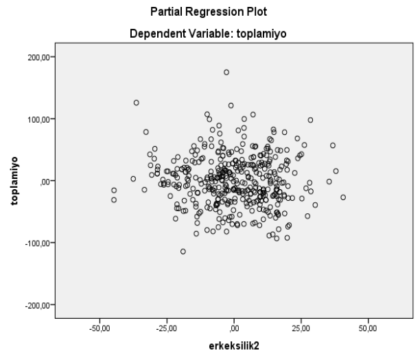
Şekil 4. Yüklemelerin bağımsız değişkenlerle ilişkileri için normallik ve doğrusallık varsayım analizi grafikleri
