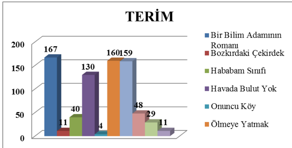
Şekil 14: Terimlerin Dağılımı
