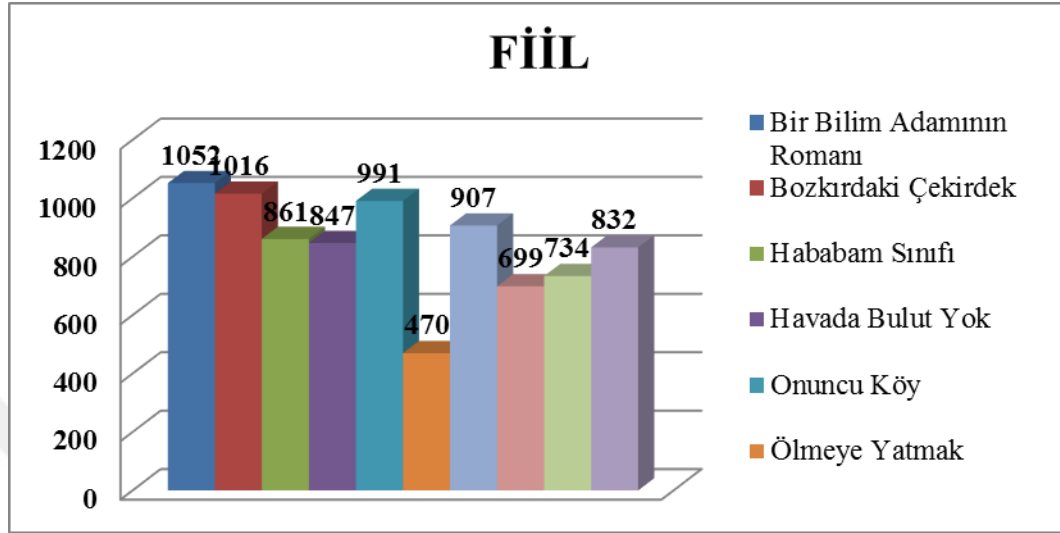
Şekil 13: Fillerin Dağılımı
