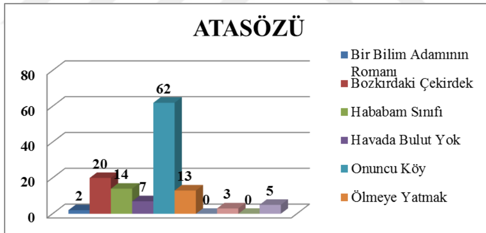
Şekil 18: Atasözlerinin Dağılımı
