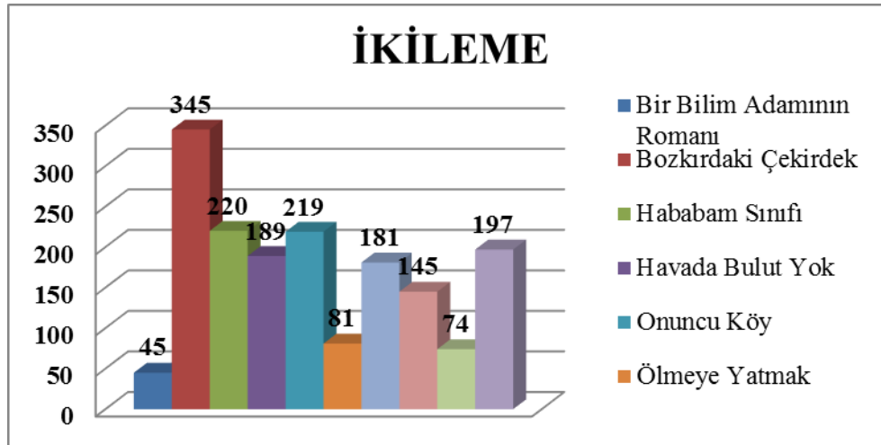
Şekil 15: İkişemelerin Dağılımı
