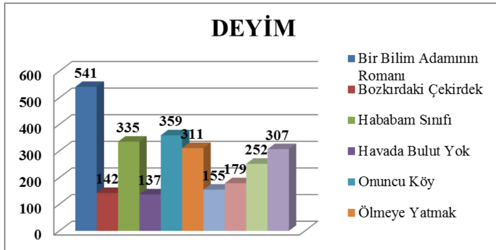
Şekil 16: Deyimlerin Dağılımı
