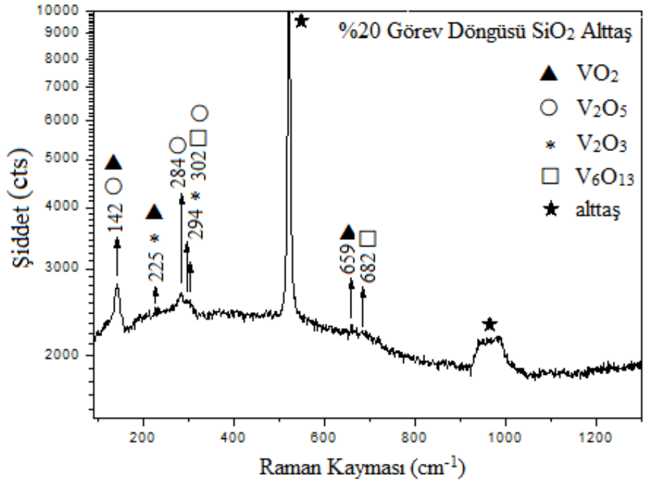
řekil 3. 23. SiO 2 alıttař zerine bytlen %20 grev dngs deęerli numune iin Raman spektrumu
