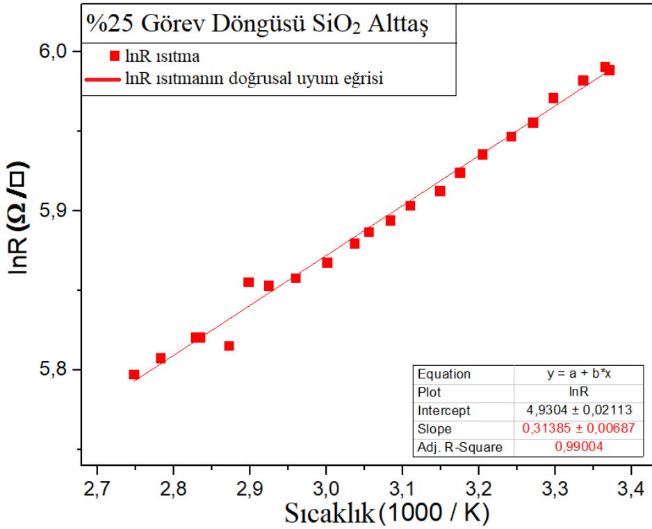
Şekil 3. 11. SiO 2 altaş üzerine büyütülen %25 görev döngüsü değerli numune için sıcaklığa bağlı lnR(1000/T) değişim eğrisi
