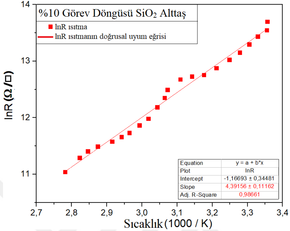
Şekil 3. 4. SiO 2 alttaş üzerine büyütülen %10 görev döngüsü değerli numune için sıcaklığa bağlı lnR(1000/T) değişim eğrisi
