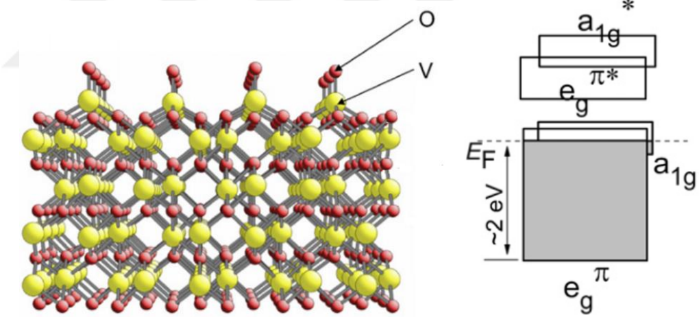
Şekil 1. 3. V_2O_3 fazının kristal yapısı[10] ve enerji band sistemi şeması [11]
