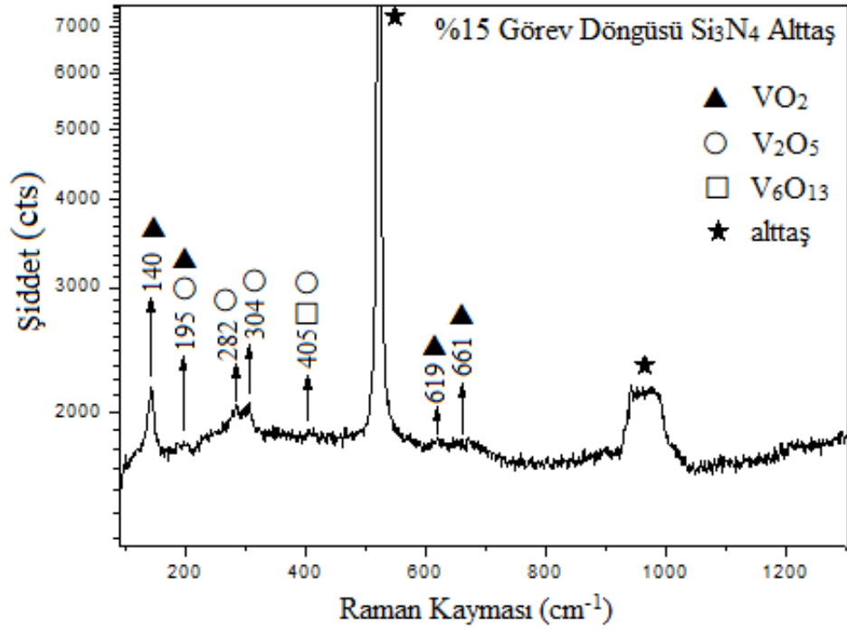
řekil 3. 22. Si 3 N 4 alıttař zerine bytlen %15 grev dngs deęerli numune iin Raman spektrumu
