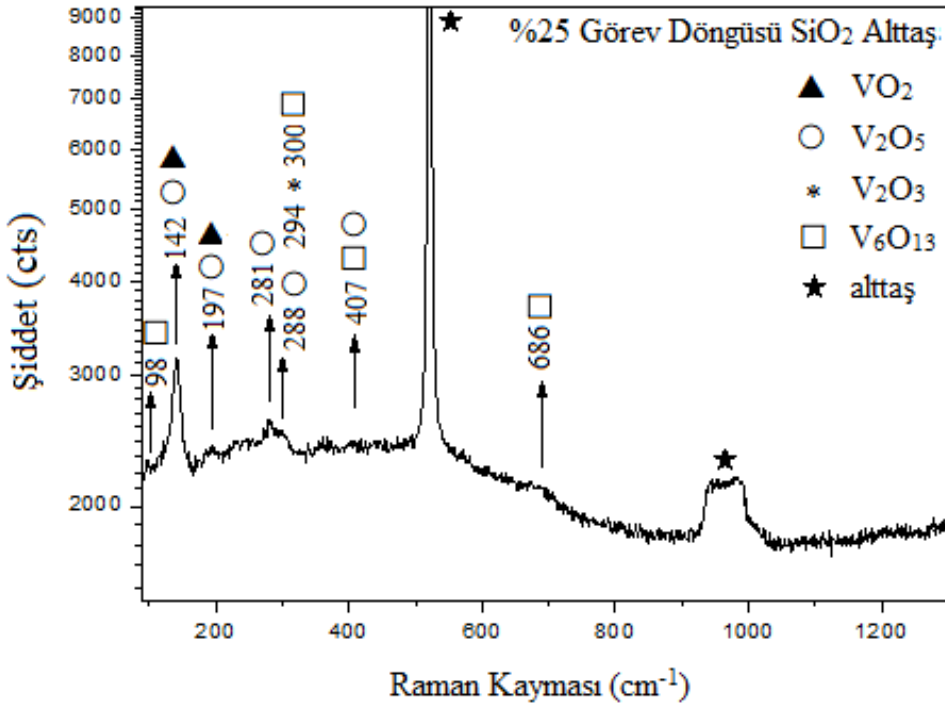
Şekil 3. 27. SiO 2 alıttař üzerine büyütölen %25 görev döngüsü deęerli numune için Raman spektrumu
