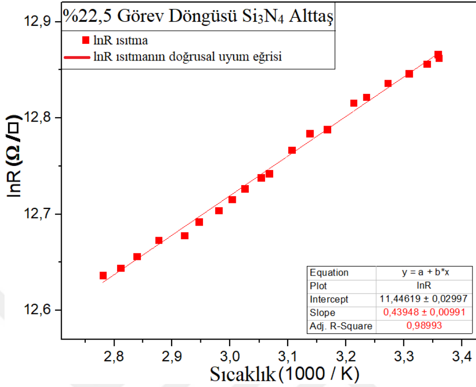
Şekil 3. 10. Si 3 N 4 altaş üzerine büyütülen %22,5 görev döngüsü değerli numune için sıcaklığa bağlı lnR(1000/T) değişim eğrisi
